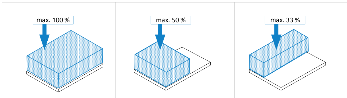
Abbildung 1: Zulässige Traglast bei Lastverteilung
