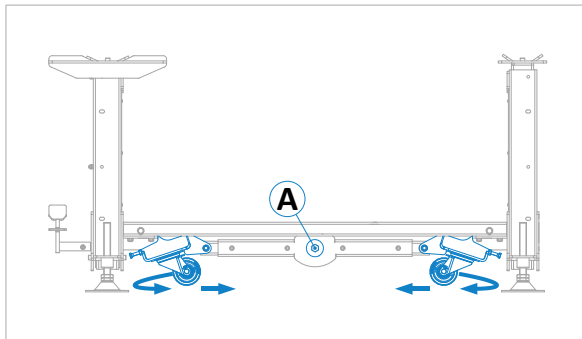
Abbildung 16: Fahrwerk ausklappen und Tisch verfahren
