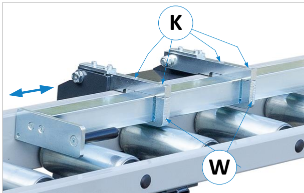
Abbildung 16: Anschlag-Nullpunkt einstellen
