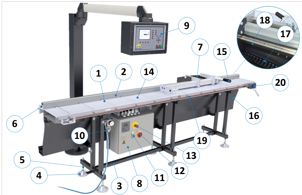
Figure 1 : convoyeur à rouleaux avec système de mesure EXAKT NC
