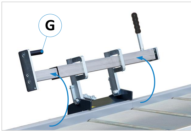
Figure 12 : rabattre la butée vers l'arrière
