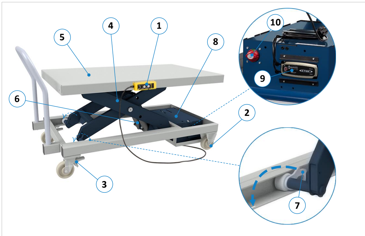
Abbildung 4: Komponenten und Bedienelemente HS 1000 | AH
