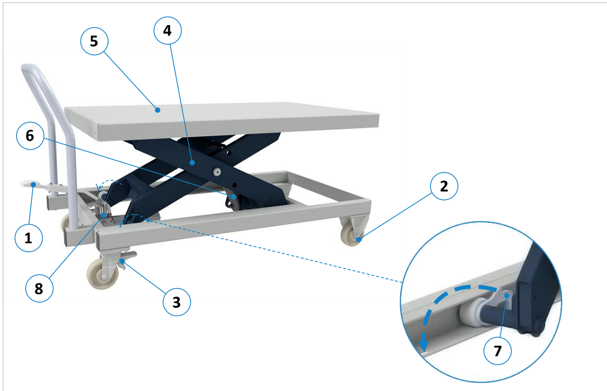
Abbildung 3: Komponenten und Bedienelemente HS 1000 | FH
