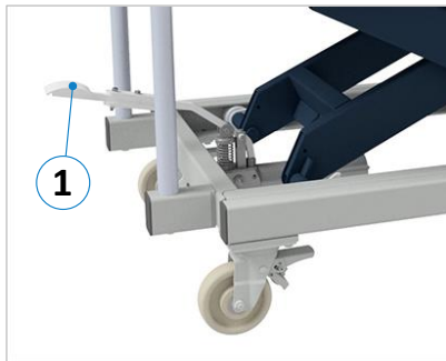
Figure 6 : pédale de réglage
