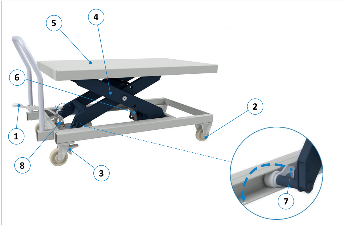
Figure 3 : composants et éléments de commande HS 1000 | FH
