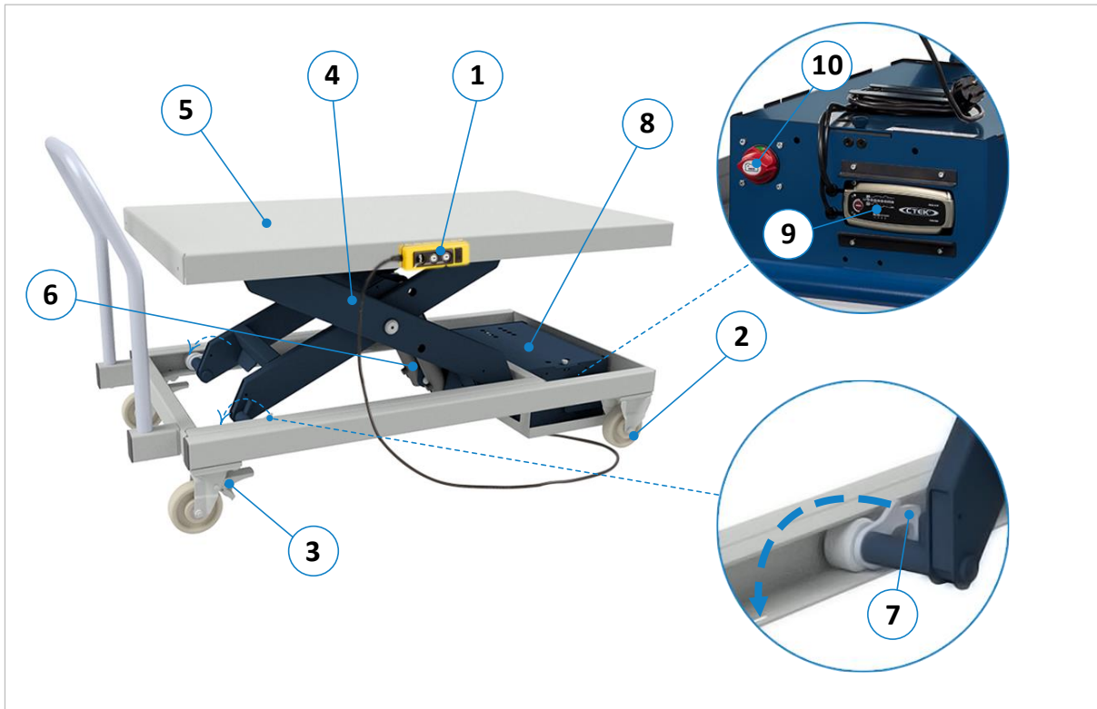
Figure 4 : composants et éléments de commande HS 1000 | AH
