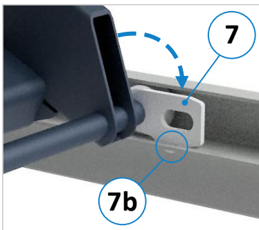
Figure 9 : cliquet d'arrêt
