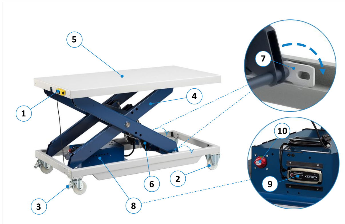
Figure 4 : composants et éléments de commande HS 1200 GRANDE | AH
