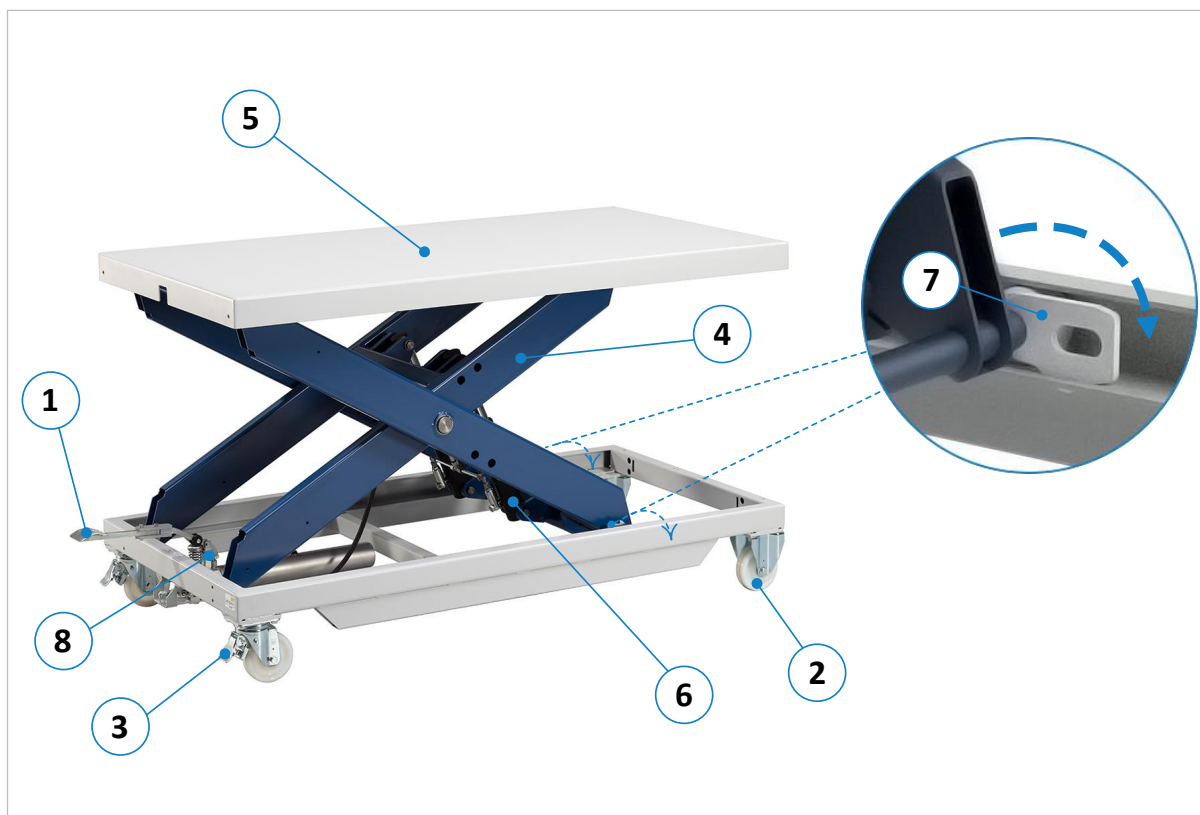
Figure 3 : composants et éléments de commande HS 1200 GRANDE | FH
