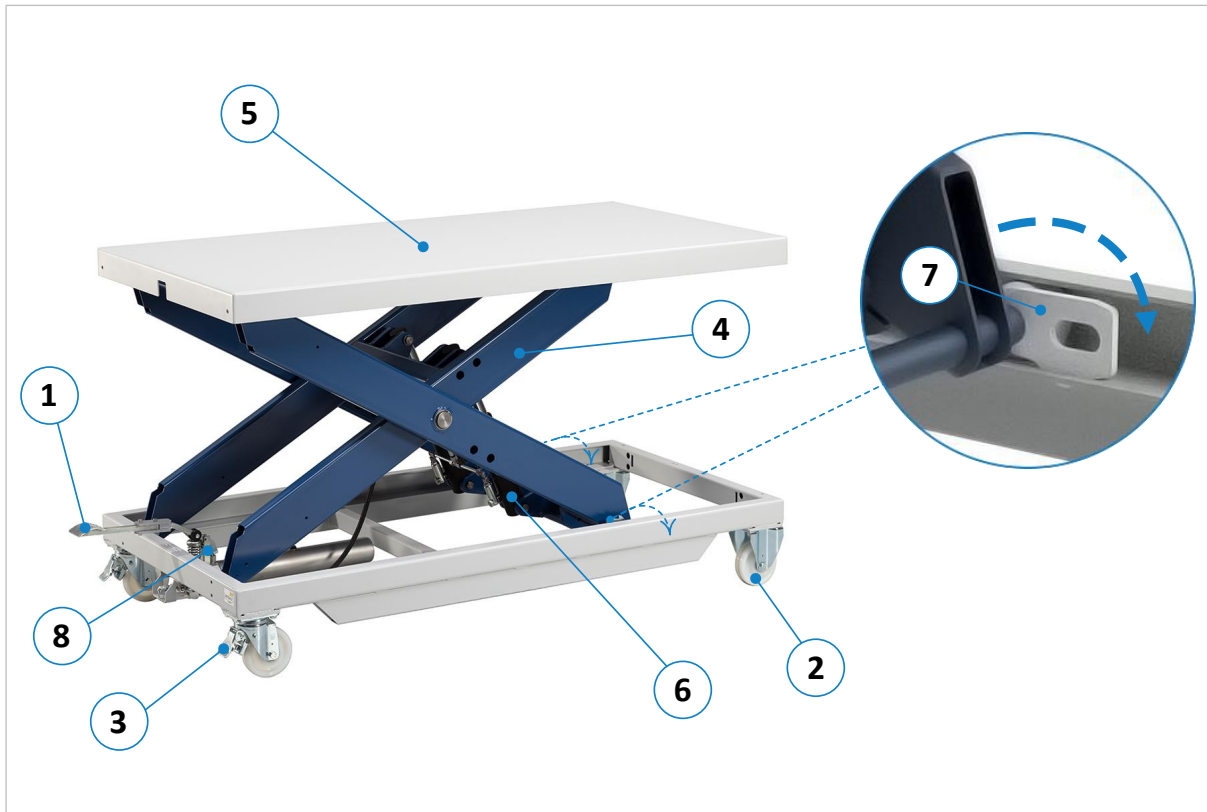
Abbildung 3: Komponenten und Bedienelemente HS 1200 GROß | FH
