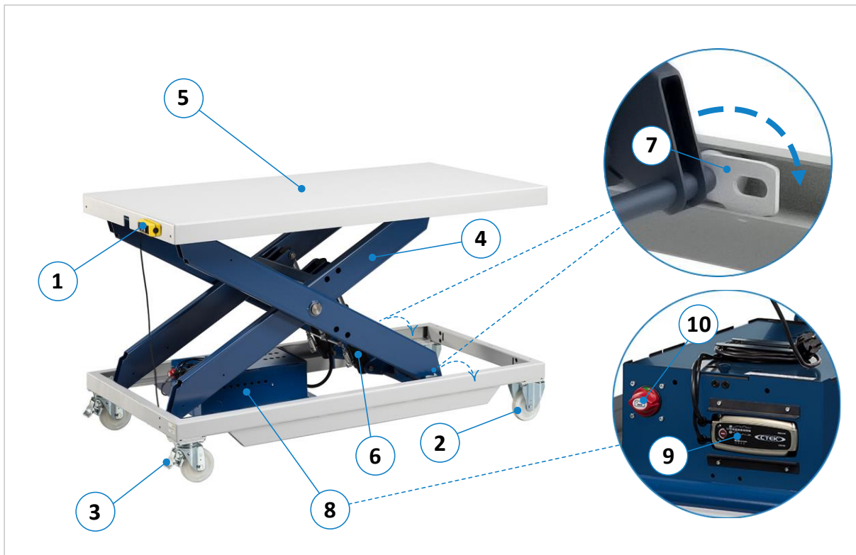
Abbildung 4: Komponenten und Bedienelemente HS 1200 GROß | AH
