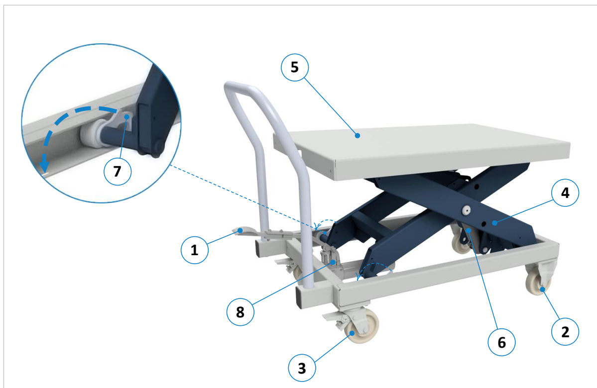
Figure 3 : composants et éléments de commande HS 1200 | FH
