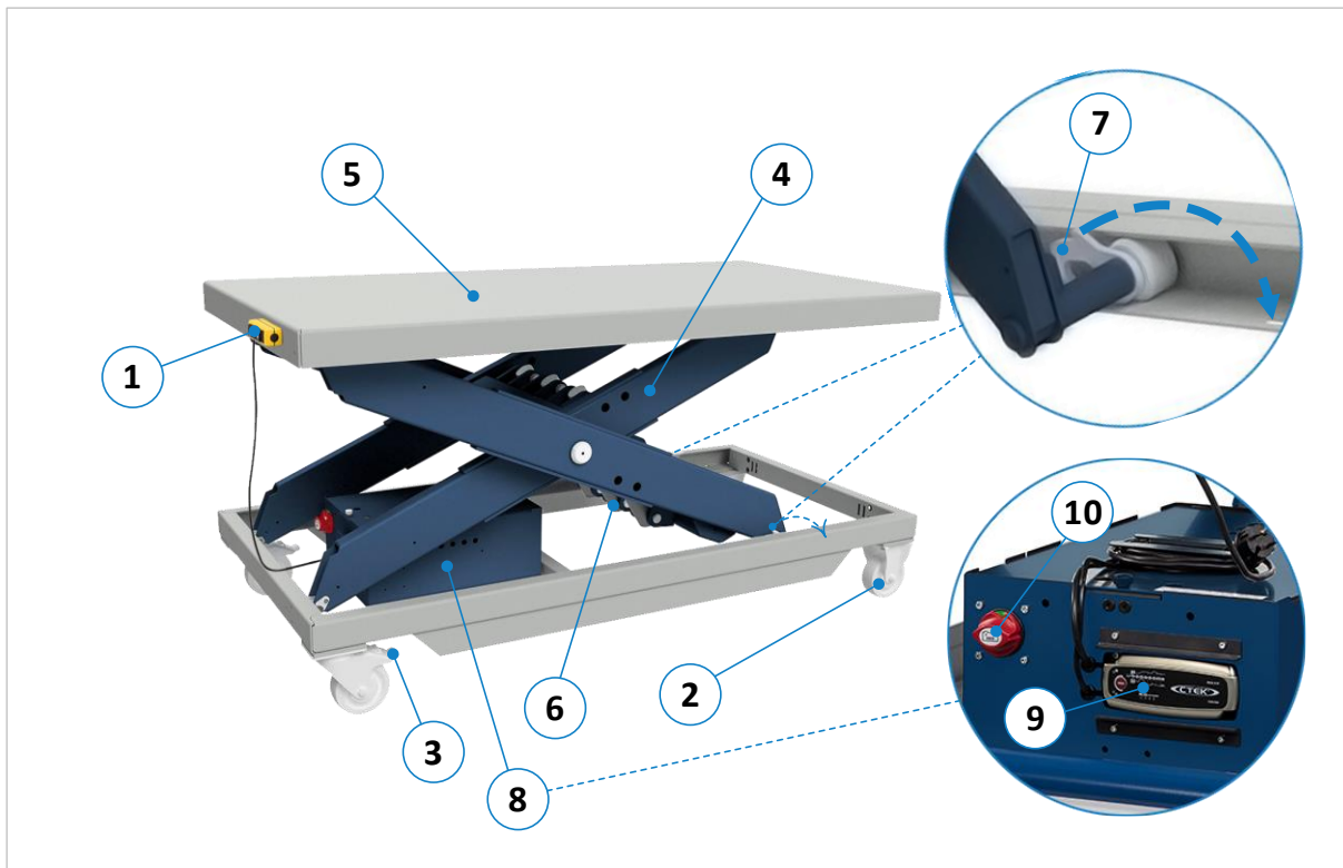
Abbildung 4: Komponenten und Bedienelemente HS 2000 GROß | AH
