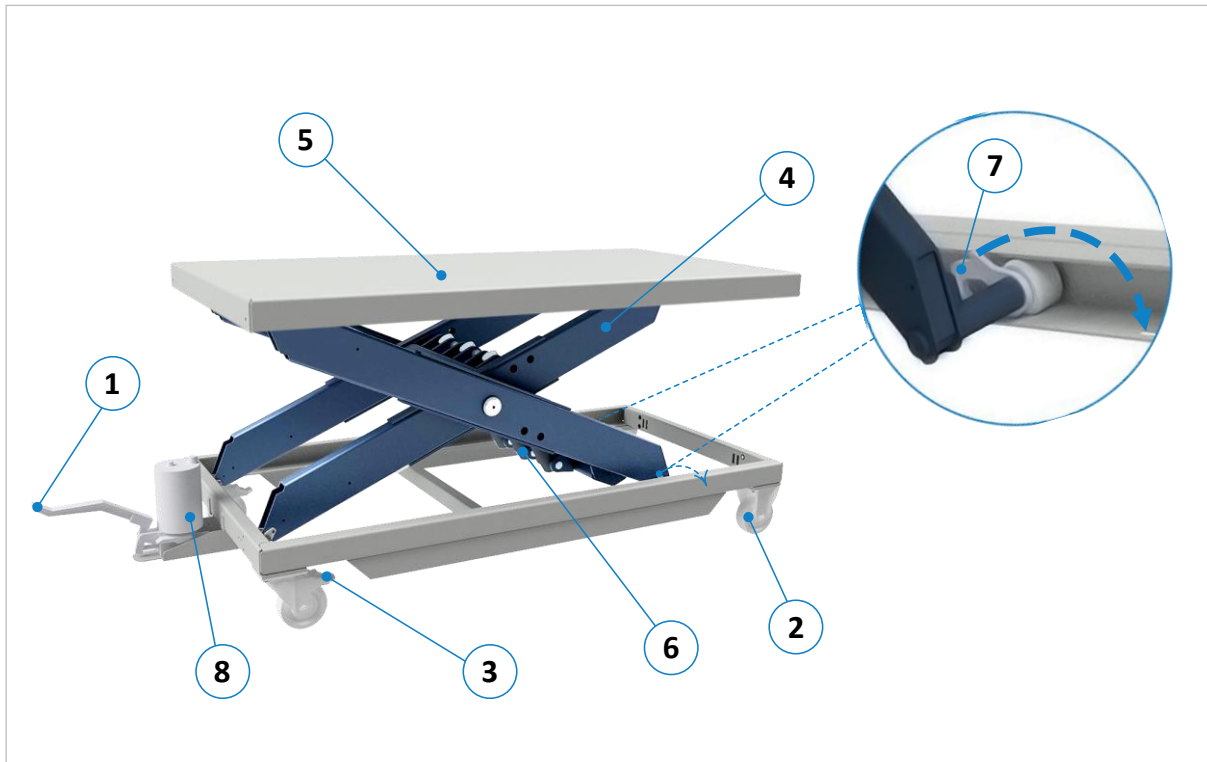
Abbildung 3: Komponenten und Bedienelemente HS 2000 GROß | FH
