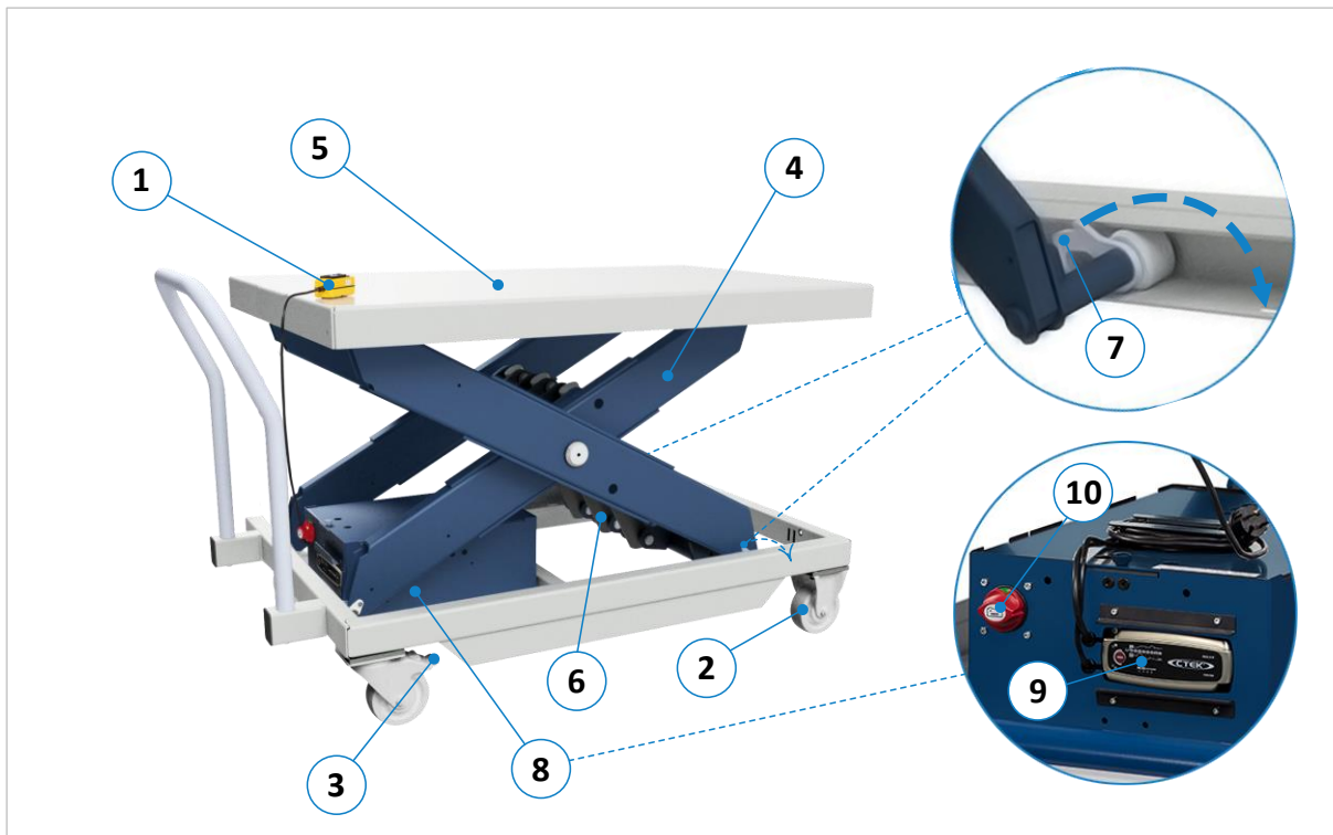
Abbildung 4: Komponenten und Bedienelemente HS 2000 | AH
