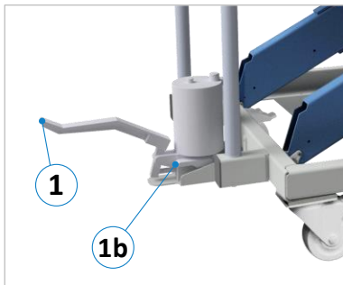
Abbildung 6: Höhenverstellung
