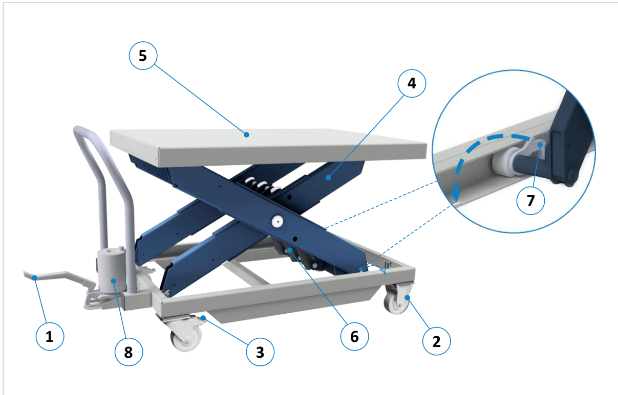
Abbildung 3: Komponenten und Bedienelemente HS 2000 | FH
