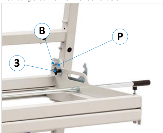
Abbildung 6: Schwenkrahmen demontieren
