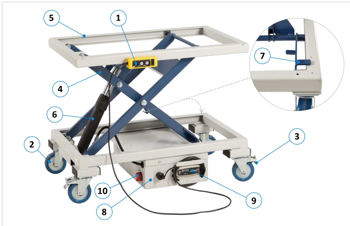
Abbildung 4: Komponenten und Bedienelemente HS 300 | AH
