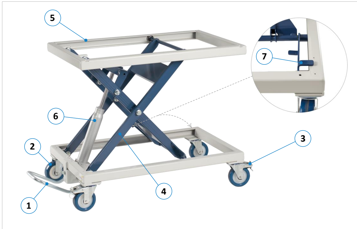
Abbildung 3: Komponenten und Bedienelemente HS 300 | FH
