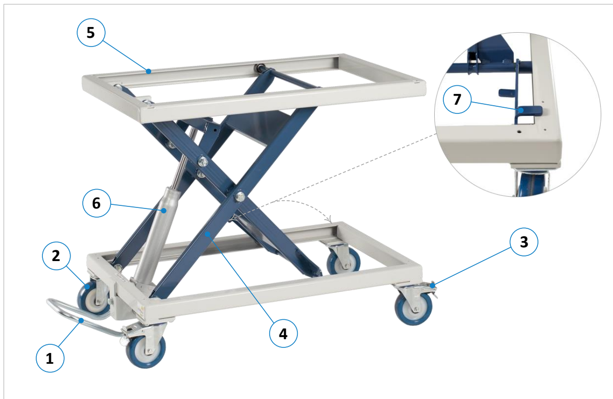
Figure 3 : composants et éléments de commande HS 300 | FH
