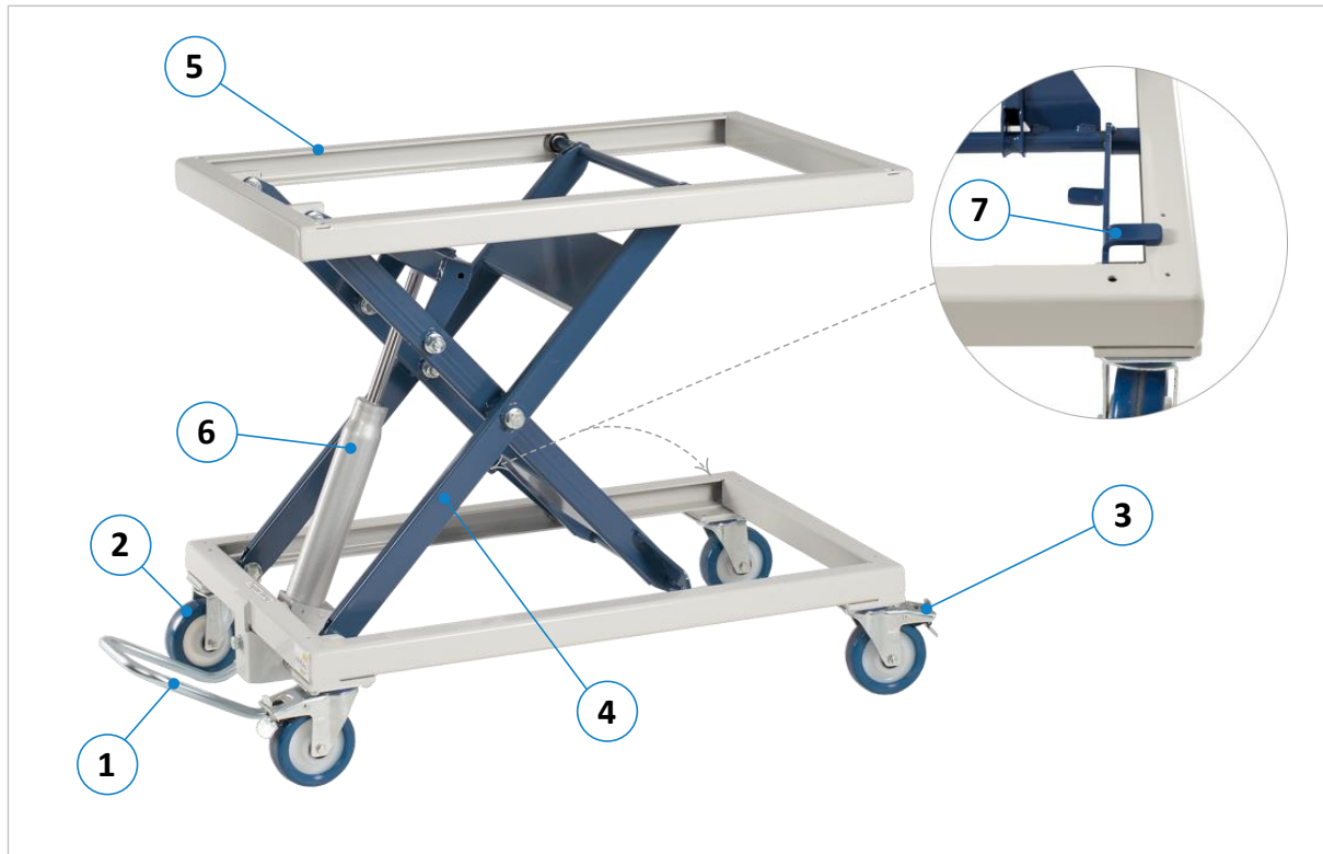
Abbildung 3: Komponenten und Bedienelemente HS 350 | FH
