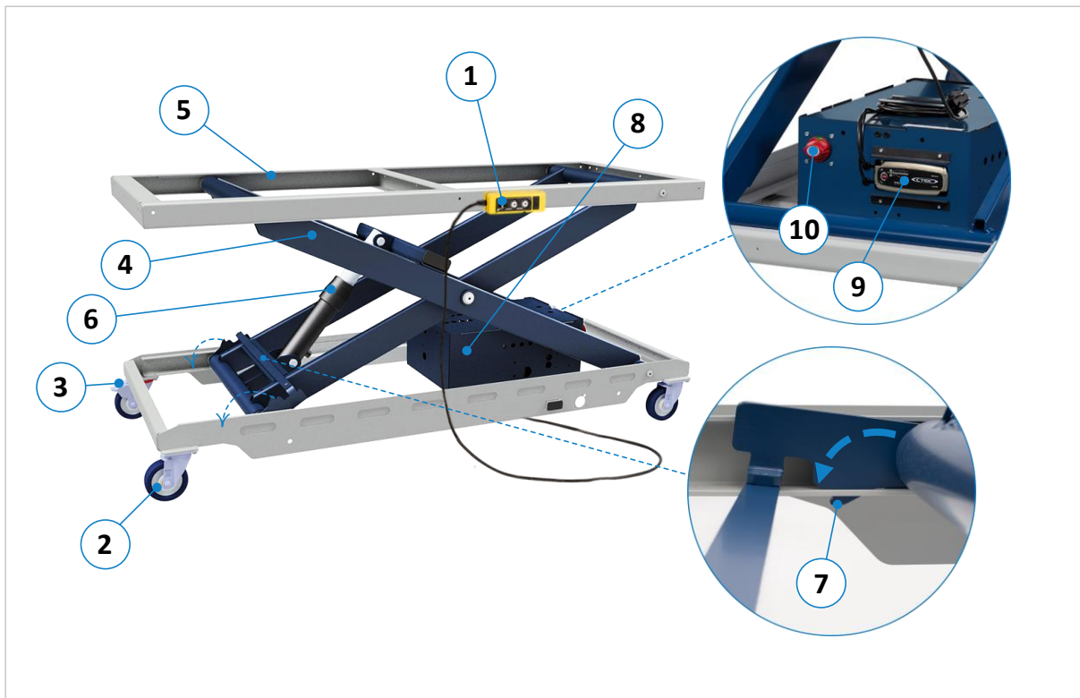
Abbildung 4: Komponenten und Bedienelemente HS 650 | AH
