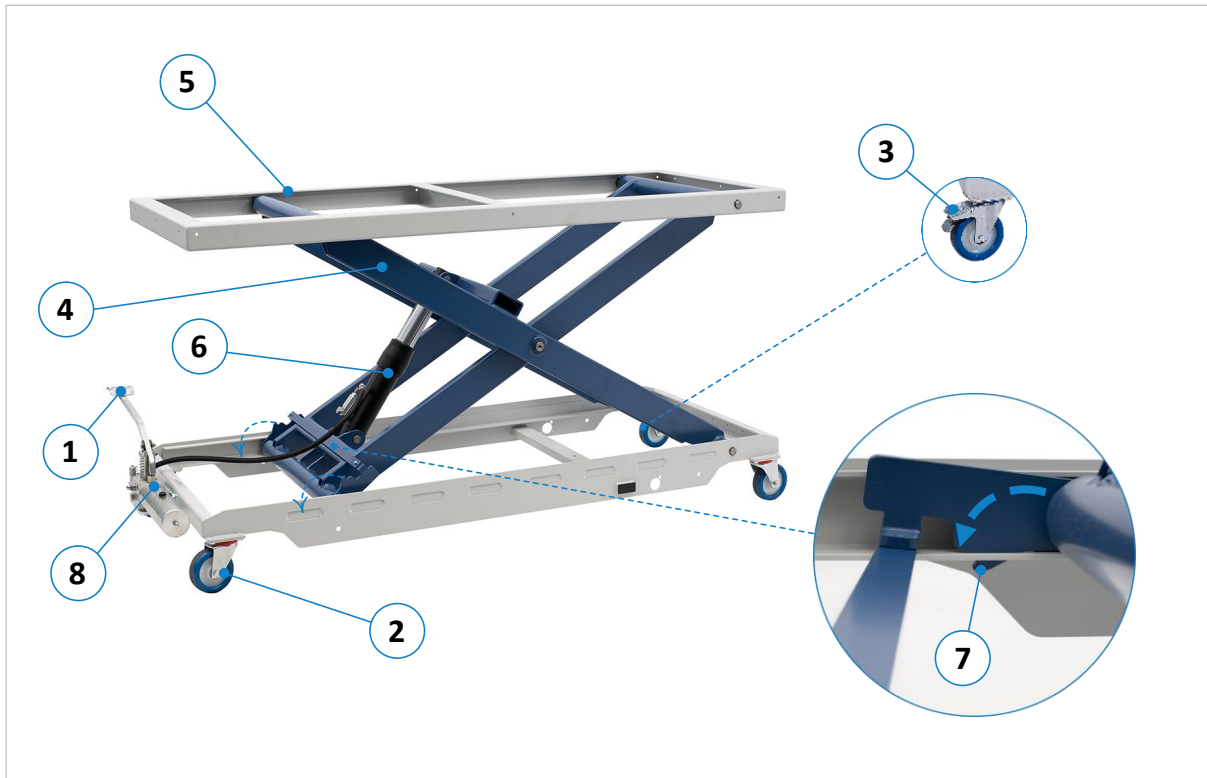
Abbildung 3: Komponenten und Bedienelemente HS 600 | FH
