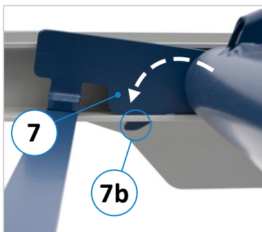
Abbildung 9: Sicherungs-Sperrklinke
