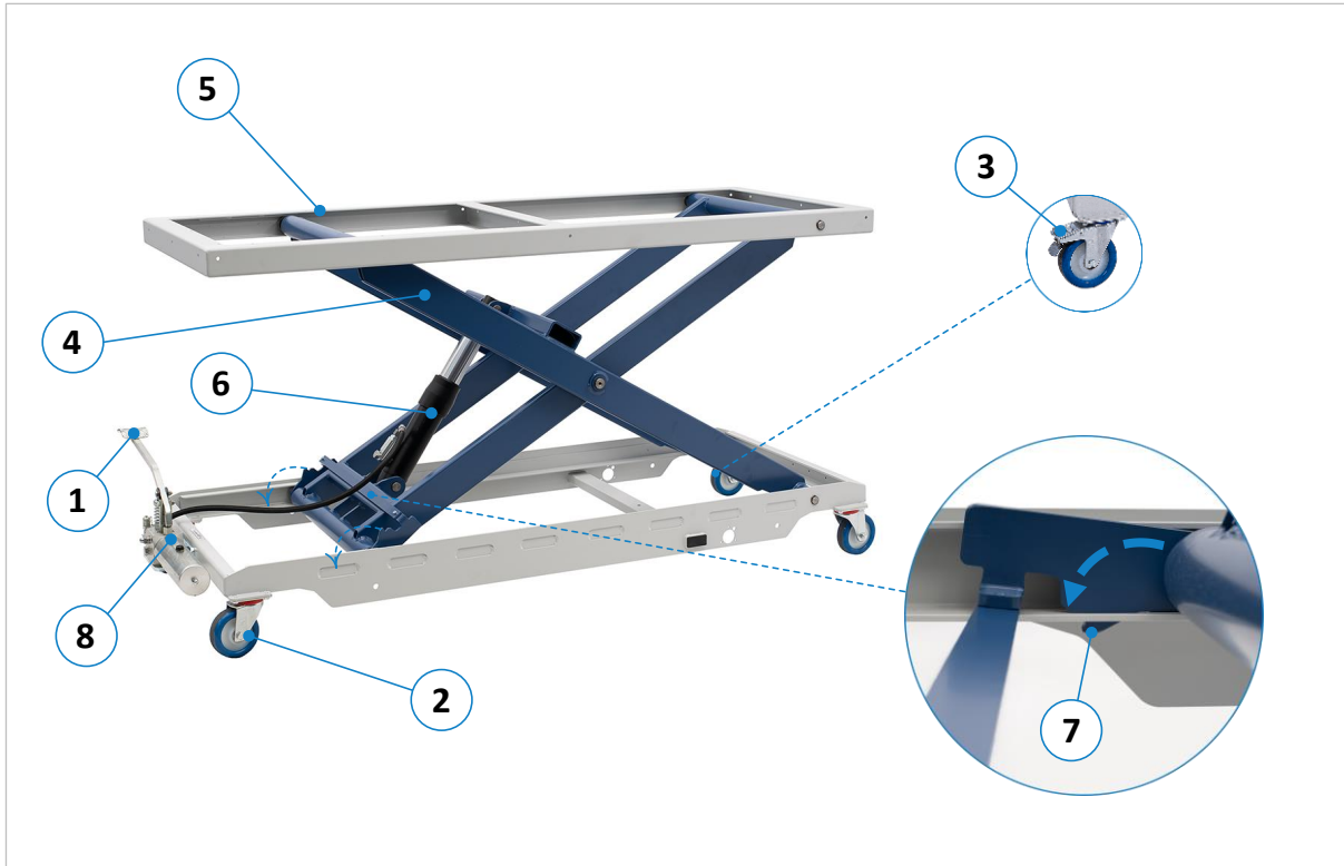
Figure 3 : composants et éléments de commande HS 600 | FH
