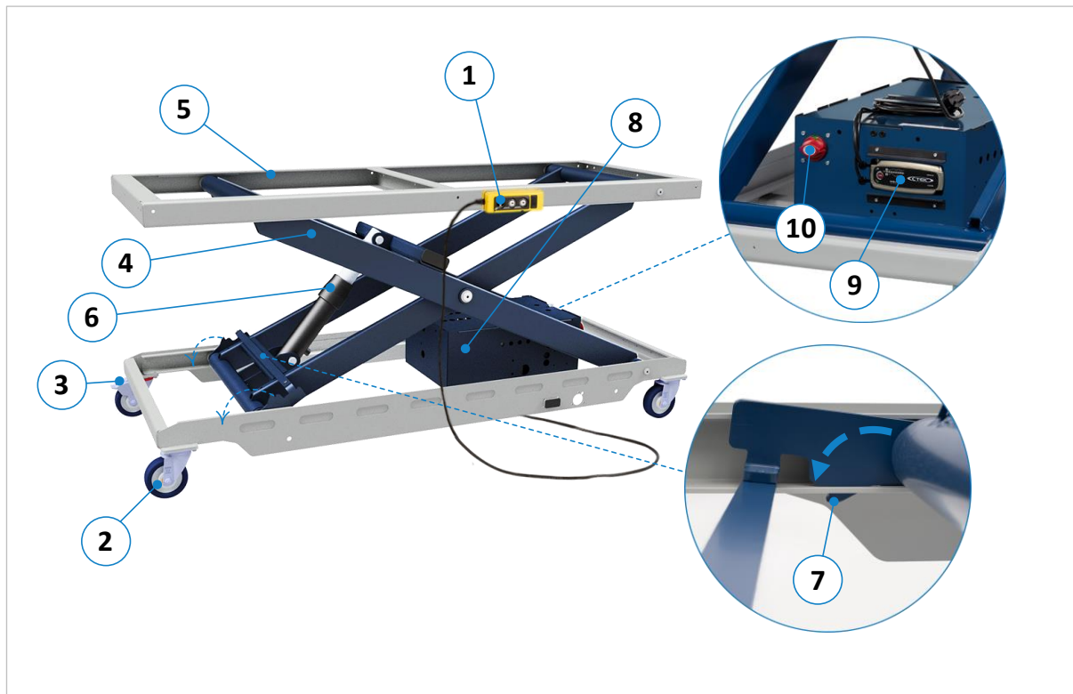
Figure 4 : composants et éléments de commande HS 600 | AH
