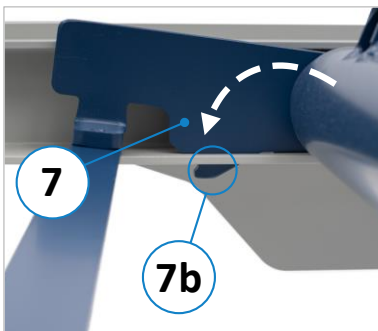
Figure 9 : cliquet d'arrêt
