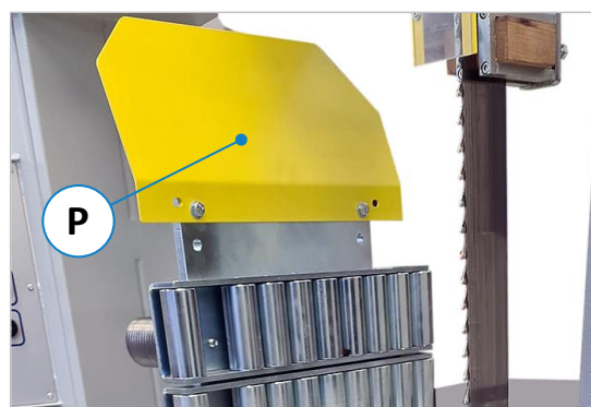
Figure 71 : protection sur la butée du rouleau
