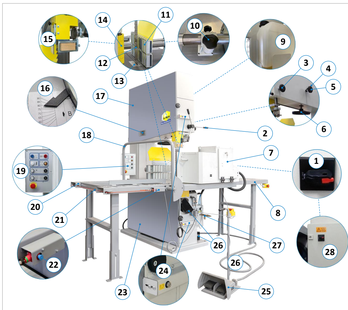
Figure 28 : composants et éléments de contrôle
