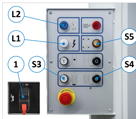
Figure 76 : interrupteur de commande pour l'avance
