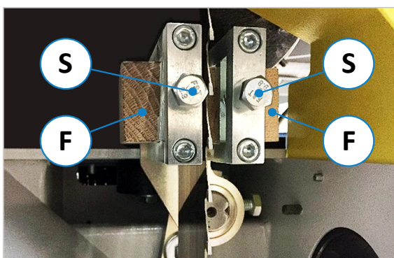
Figure 62 : guide inférieure de la lame de scie
