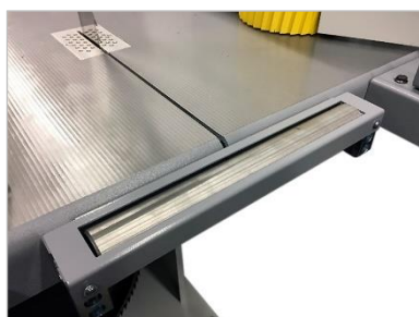
Figure 47 : rouleau de table monté
