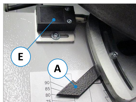
Figure 68 : interrupteur de fin de course (E)
