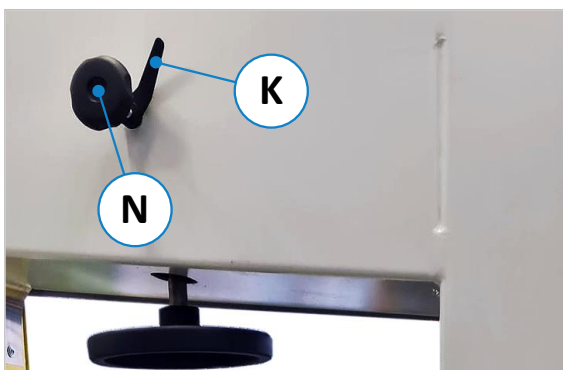
Figure 60 : corriger l'inclinaison de la lame de scie
