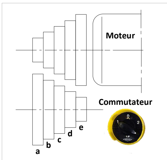
Figure 79 : couches de courroies pour la vitesse d'avance
