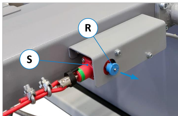
Figure 39 : réinitialiser l'état d'arrêt d'urgence
