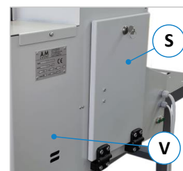
Figure 22 : unité d'avance
