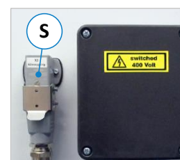
Figure 20 : connecteur
