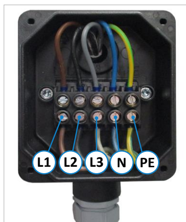
Figure 16 : boîte à bornes
