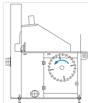
Figure 17 : sens de rotation
