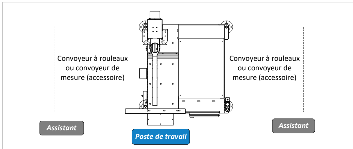
Figure 15 : positions de travail (vue de dessus)
