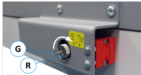
Figure 26 : interrupteur de sécurité - porte déverrouillée
