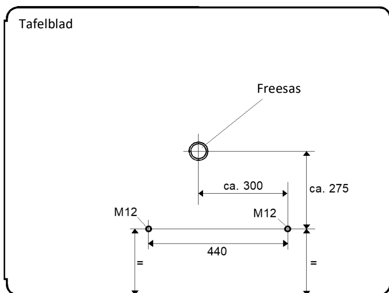
Figuur 55: Boorschets - Aanpassen van pen- en groefbevestiging
