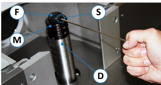
Figuur 14: Freeshouder met snelspanner
