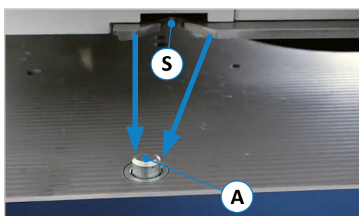
Figuur 26: Opening op slotbout uitlijnen
