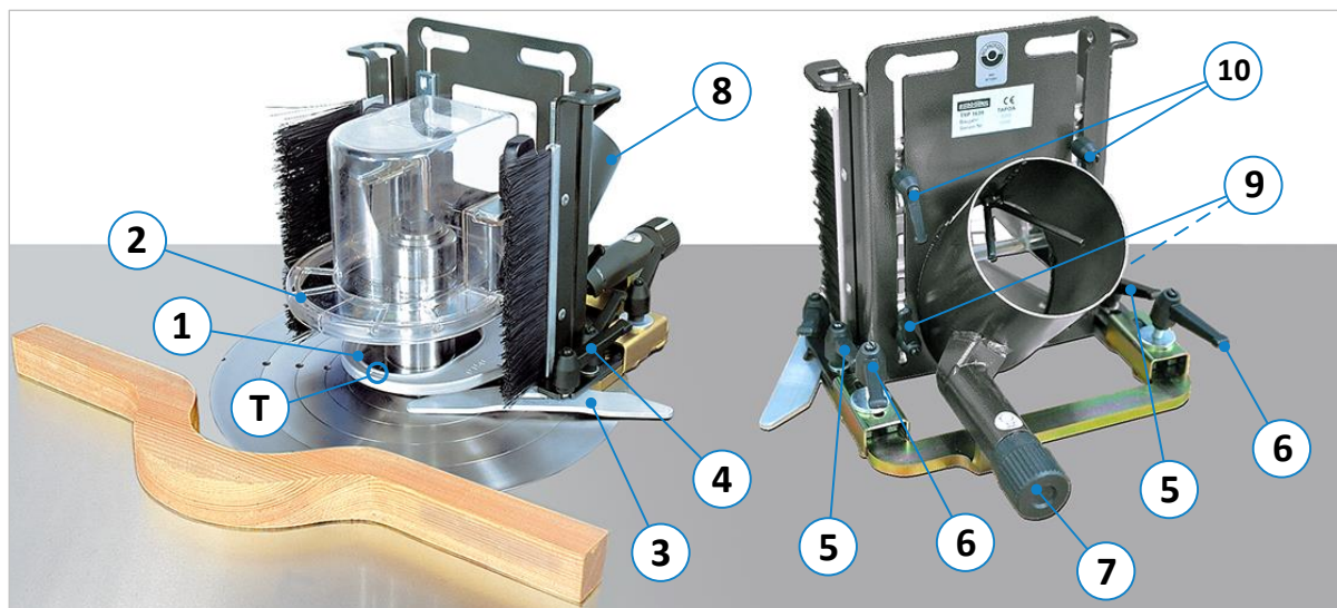
Figuur 40: Bedienungselementen van de TAPOA 1639 gebogen afrastering
