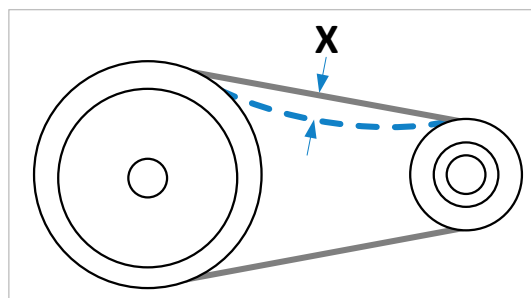
Figuur 66: Controleer de riemspanning
