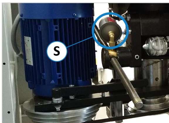
Figuur 67: Vervang het smeertoestel
