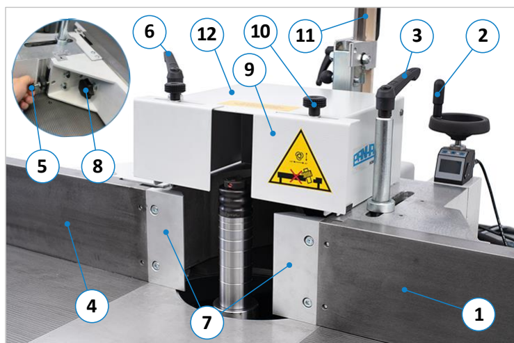
Figuur 28: Bedienungselementen aanslag type 301
