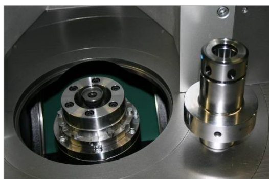
Figuur 21: Losse klemcassette met freeshouder
