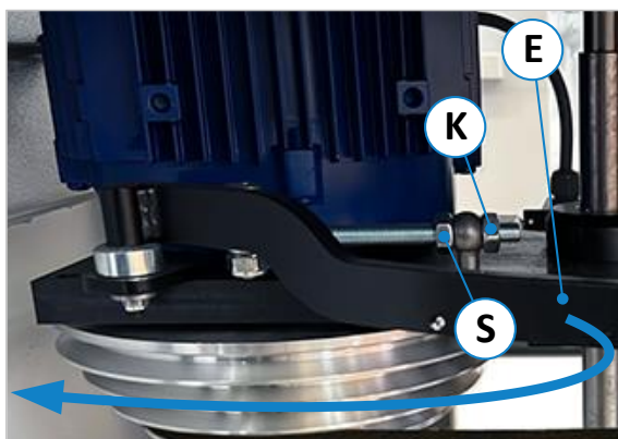
Figuur 64: Spanriem (245|100)
