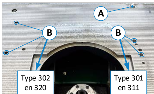
Figuur 24: Borgbouten en borggaten
