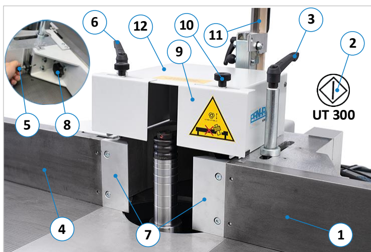
Figuur 35: Bedieningselementen Aanslag type 311
