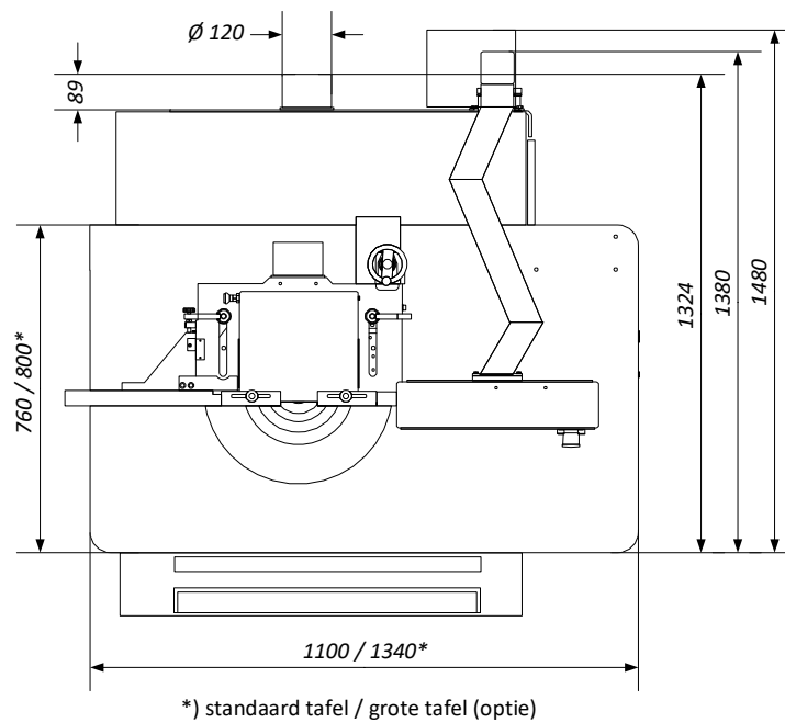
Figuur 4: Afmetingen zonder tafelverlengingen
