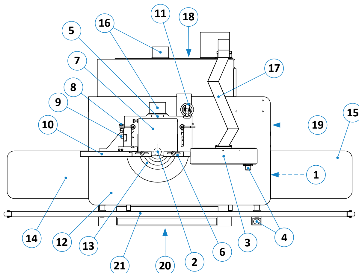
Figuur 11: Componenten en controles
