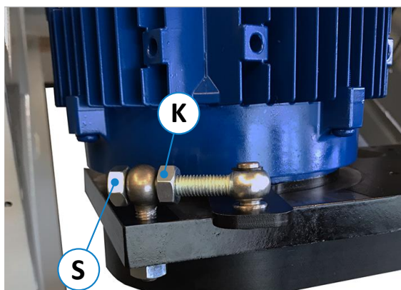
Figuur 65: Spanriem (245|200 en 245|300)
