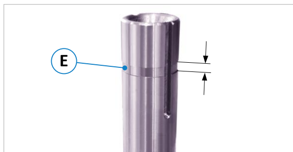
Figuur 15: Markering voor bovenste afstandsring
