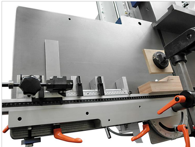
Figuur 57: Lengte-aanslag LAS-M
