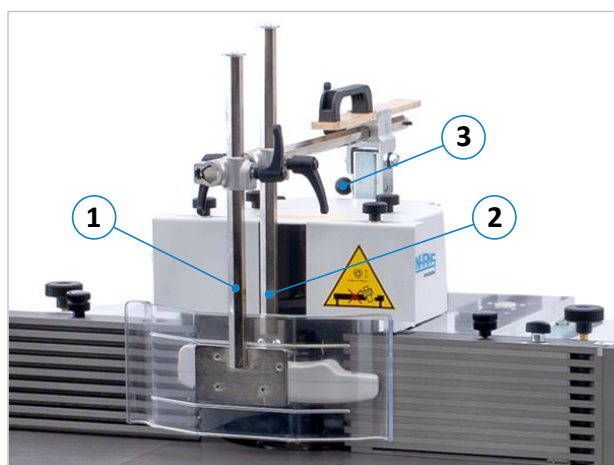
Figuur 42: Freesbeveiliging 1629 GAMMA V
