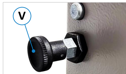
Figuur 29: Vergrendelbout type 301
