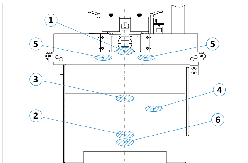
Figuur 69: Smeerpunten op de machine
