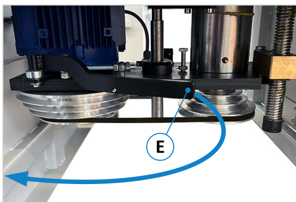
Figuur 22: Hendel om de riem los te maken
