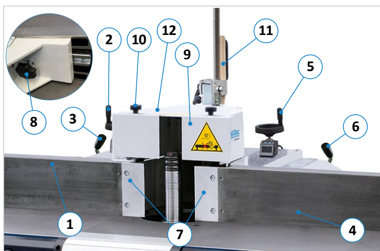
Figuur 30: Bedieningselementen aanslag type 302
