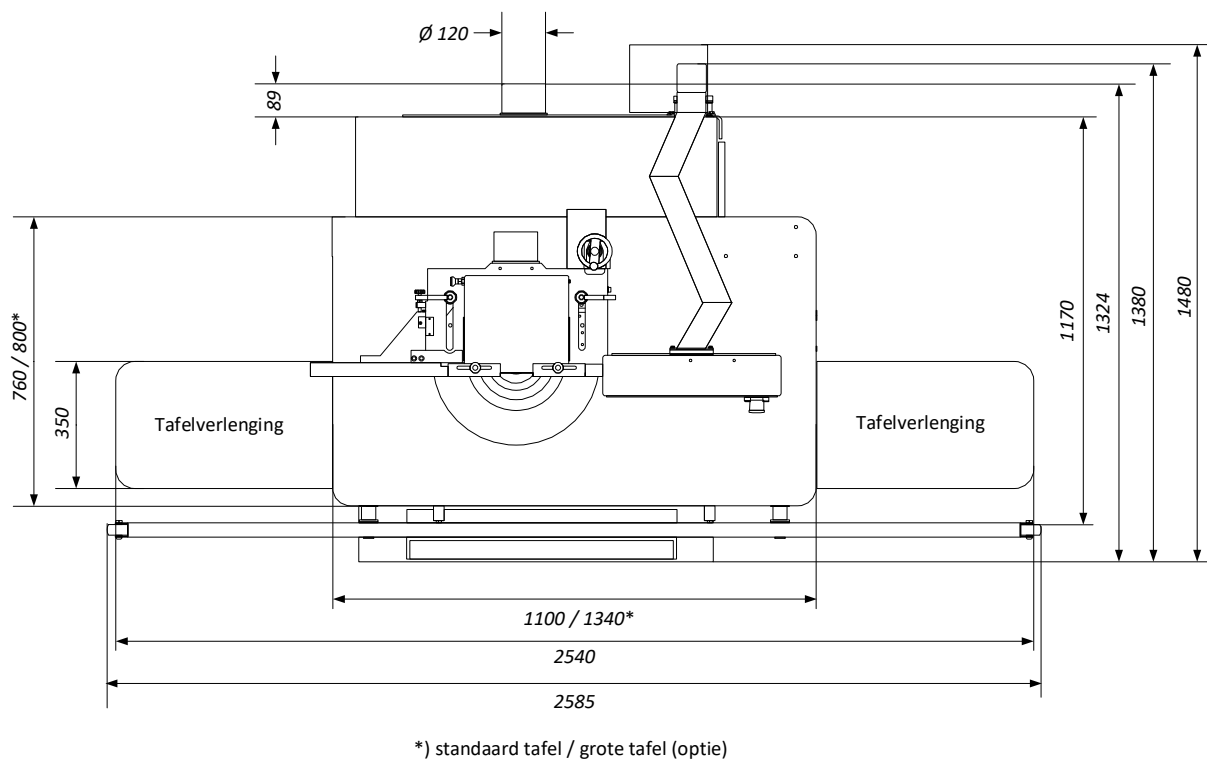
Figuur 5: Afmetingen met optionele tafelverlengingen
