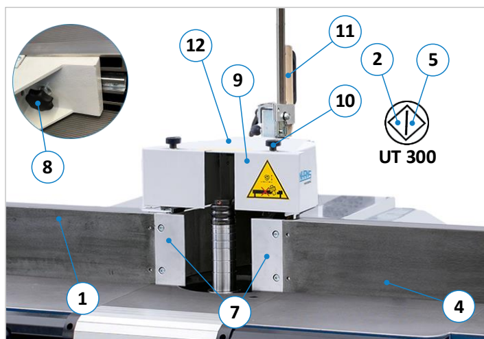
Figuur 37: Bedieningselementen aanslag type 320
