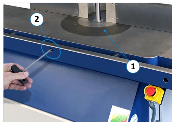
Figuur 49: Draaischijf en opening voor klemming
