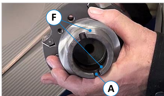
Figuur 19: Klemvlakken en vergrendeling
