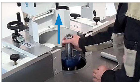
Figuur 18: Freeshouder verwijderen
