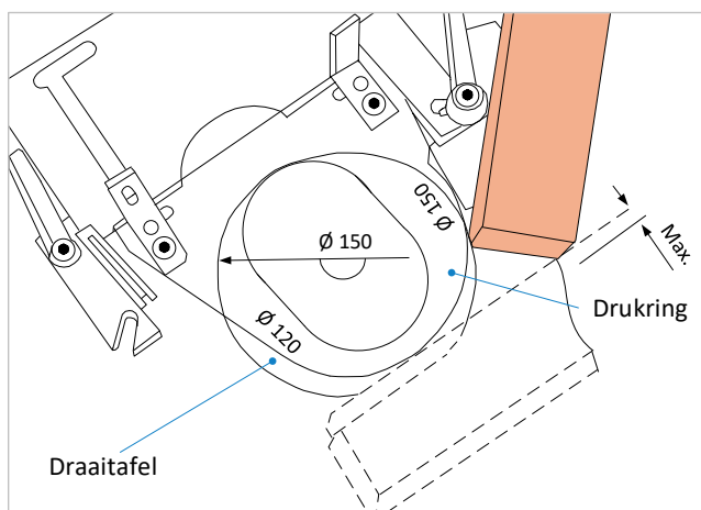
Figuur 41: Afstellen van de TAPOA 1639 bogenfreesaanslag
