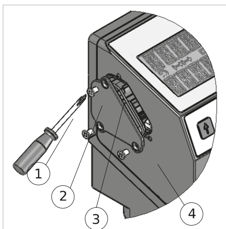
Figuur 34: Handwiel batterij vervangen
