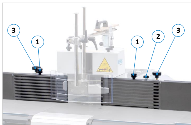
Figuur 45: Bedieningselementen Integrale aanslagplaten
