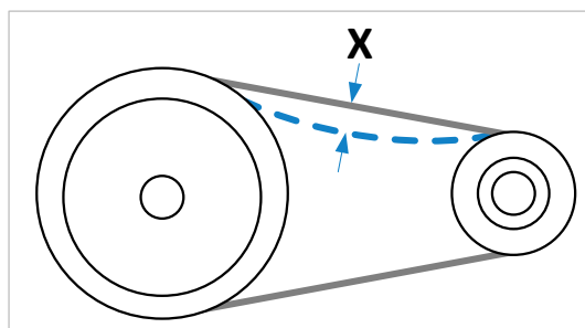
Figuur 51: Controleer de riemspanning
