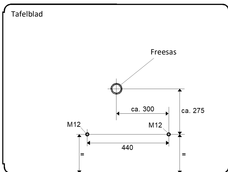
Figuur 44: Boorschets - Aanpassen van pen- en groefbevestiging
