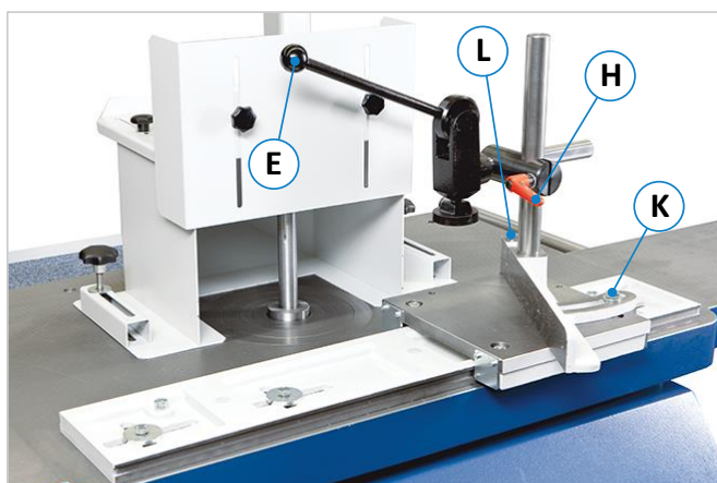
Figuur 42: Pen- en groefmachine 1376
