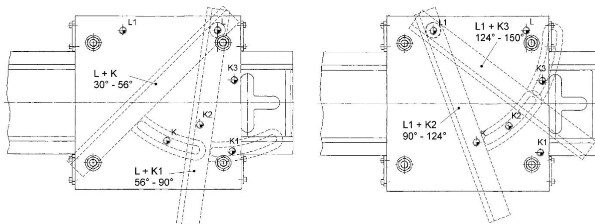
Figuur 43: Instelbare hoeken (positie van de schroeven)
