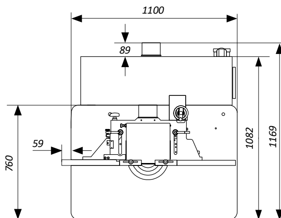
Figuur 4: Afmetingen - bovenaanzicht 1
