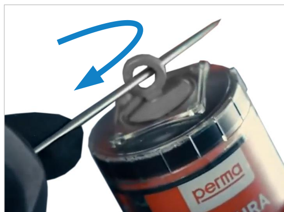
Figuur 53: Activering met ringoog
