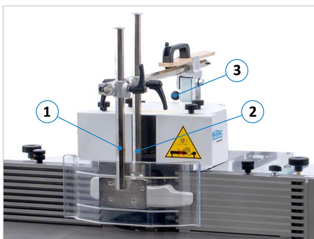
Figuur 33: Freesbeveiliging 1629 GAMMA V
