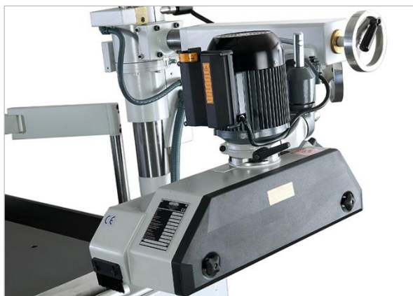
Figuur 46: Aanvoerapparaat type PV84
