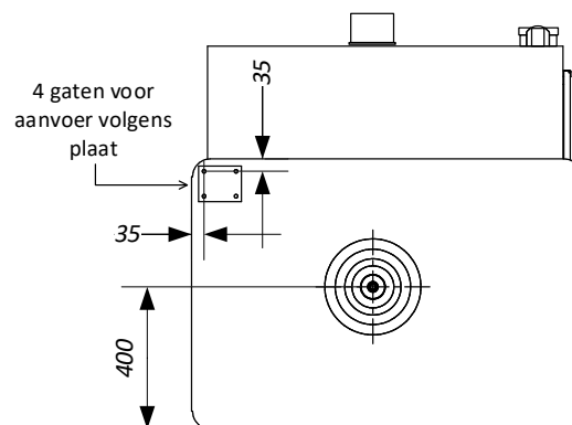
Figuur 5: Afmetingen - bovenaanzicht 2
