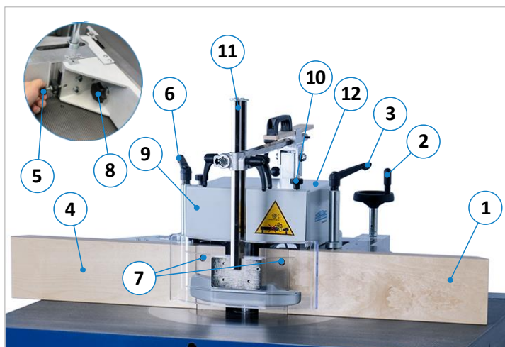
Figuur 25: Bedieningselementen aanslag type 215
