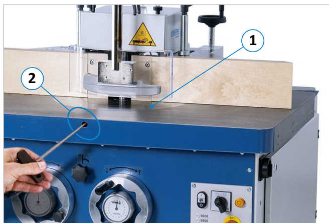
Figuur 39: Draaischijf en opening voor klemming
