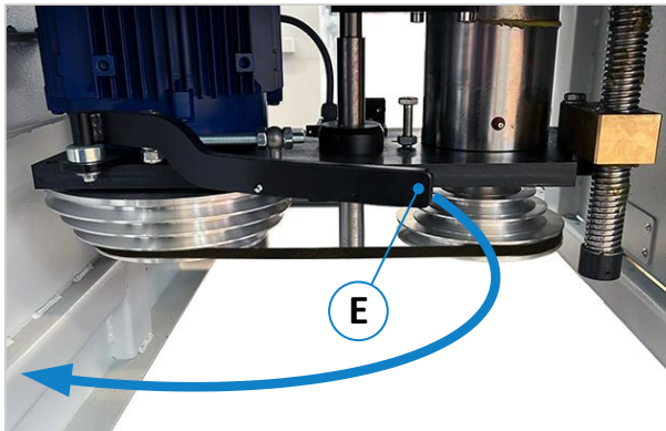
Figuur 16: Hendel om de riem los te maken
