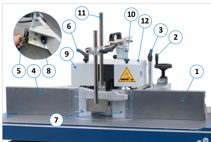
Figuur 26: Bedieningselementen aanslag type 216
