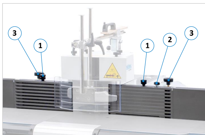
Figuur 36: Bedieningselementen Integrale aanslagplaten
