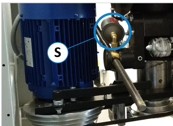
Figuur 52: Vervang het smeertoestel
