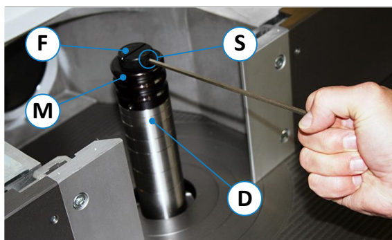
Figuur 18: Freeshouder met snelspanner
