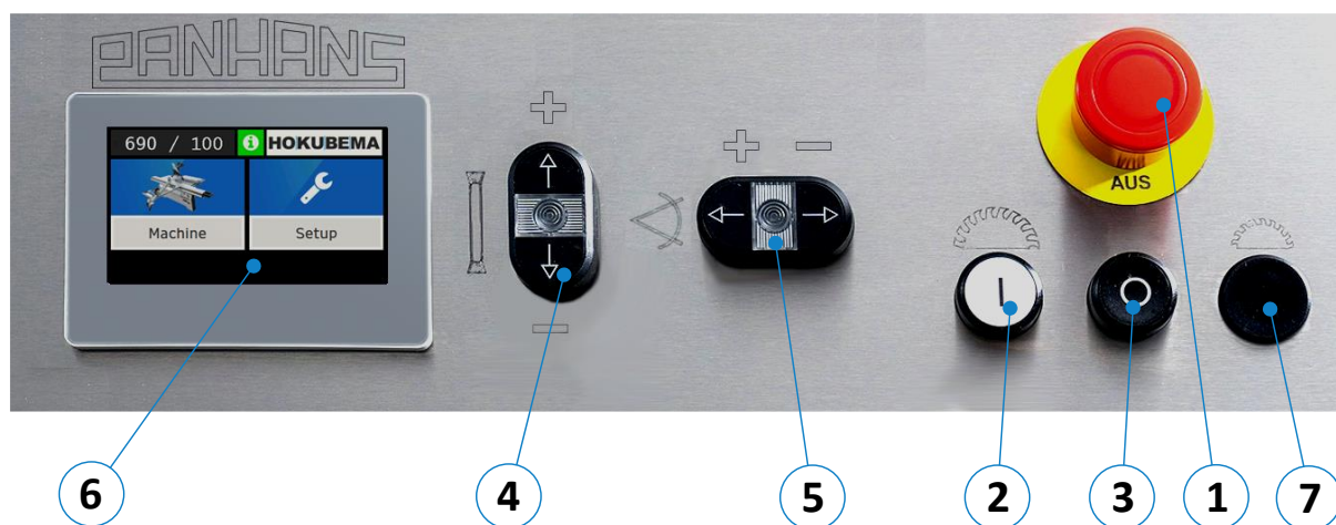
Figure 28 : éléments de commande
