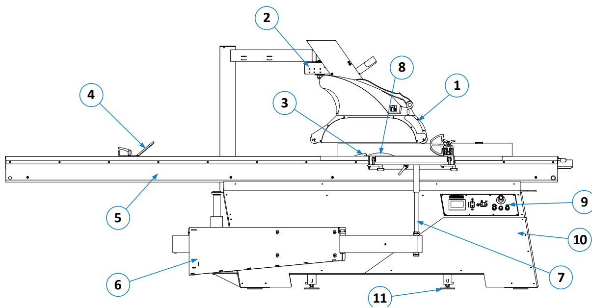
Figure 17 : composants et éléments de commande - vue de face
