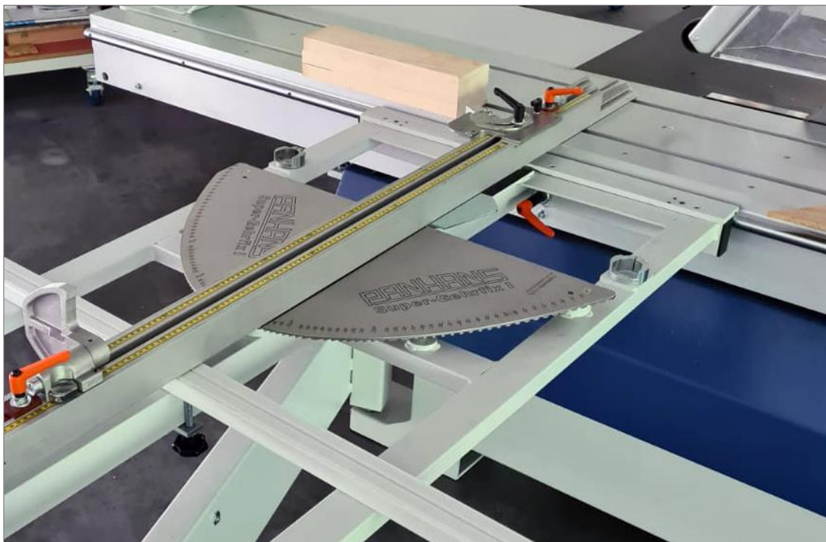
Figure 59 : guide à onglets et de longueur „Super-Gehrfix I“
