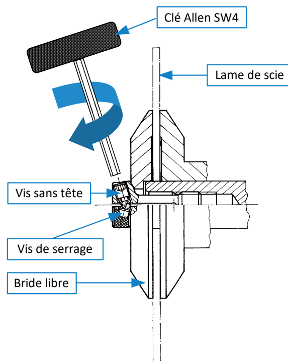
Figure 48 : bride de la lame de scie
