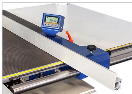
Figure 68 : guide parallèle avec « Digit PAB »
