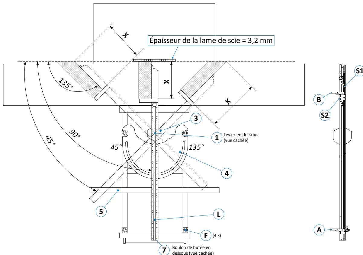
Figure 63 : aperçu et éléments de commande
