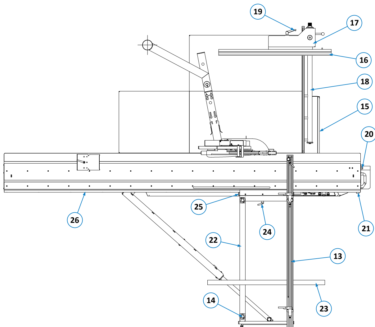
Figure 18 : composants et éléments de commande - vue de dessus
