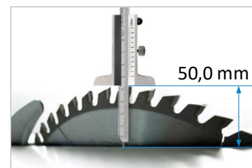
Figure 36 : hauteur de la lame 50 mm
