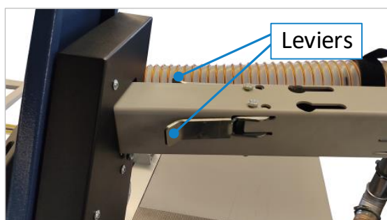
Figure 26 : bras pivotant pour capot de protection
