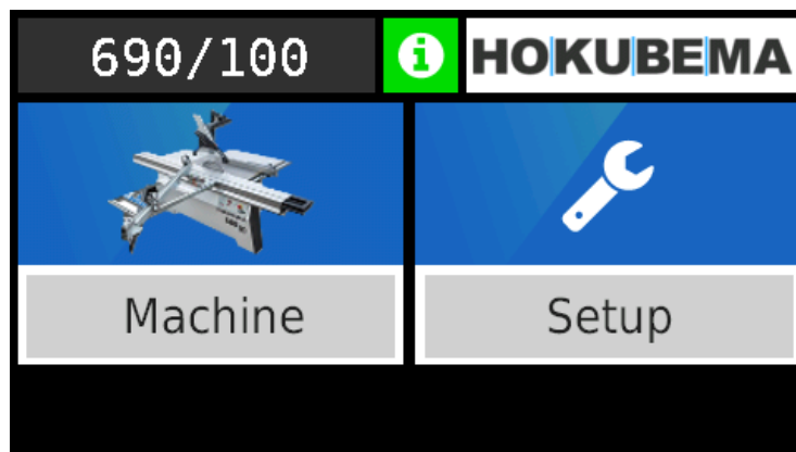
Figure 32 : écran d'accueil
