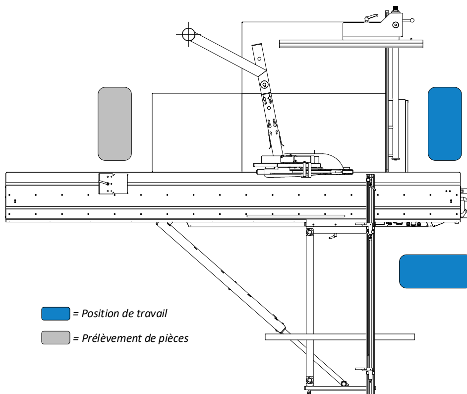
Figure 7 : postes de travail
