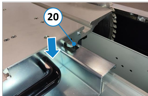
Figure 46 : cliquet de sécurité sur la table coulissante
