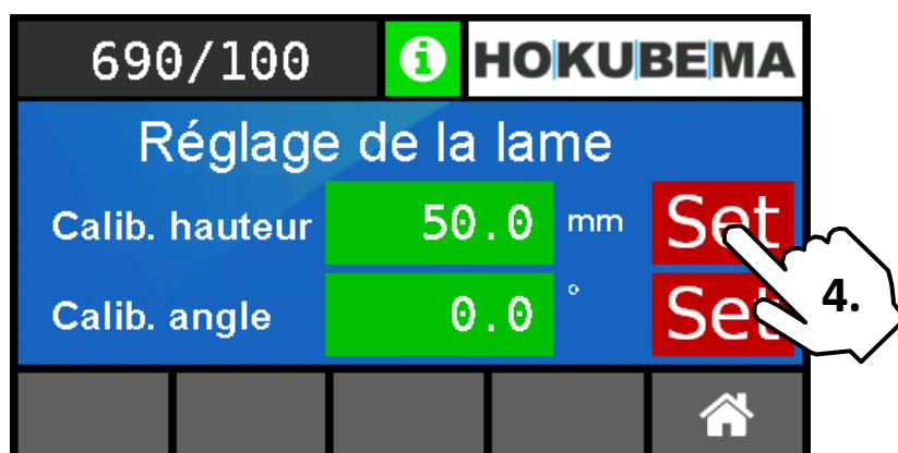
Figure 38 : reprendre la valeur de calibrage pour la hauteur
