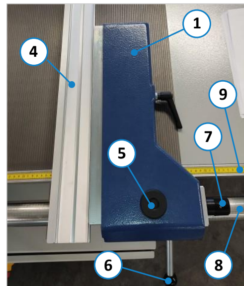
Figure 22 : utilisation du guide parallèle
