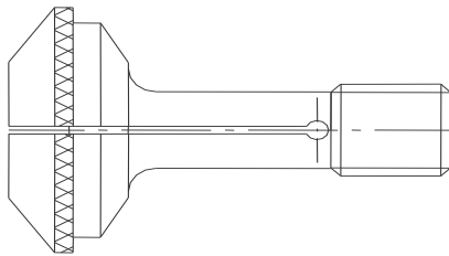
Figure 72 : vis de serrage rapide « Quickstep »
