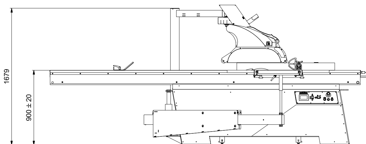
Figure 8 : dimensions (vue de face)
