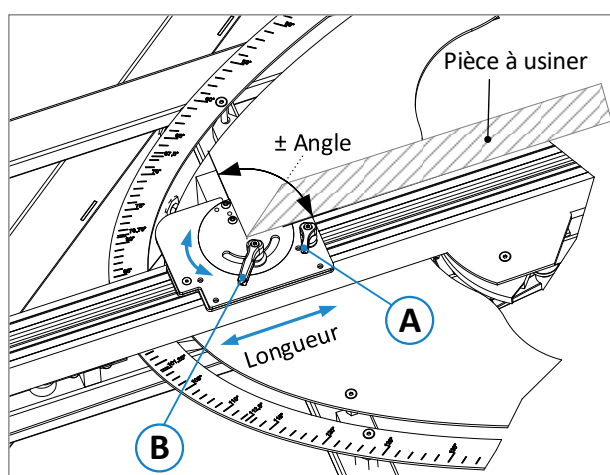
Figure 65 : utilisation du guide d'onglet auxiliaire
