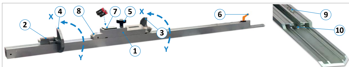
Figure 52 : - guide télescopique
