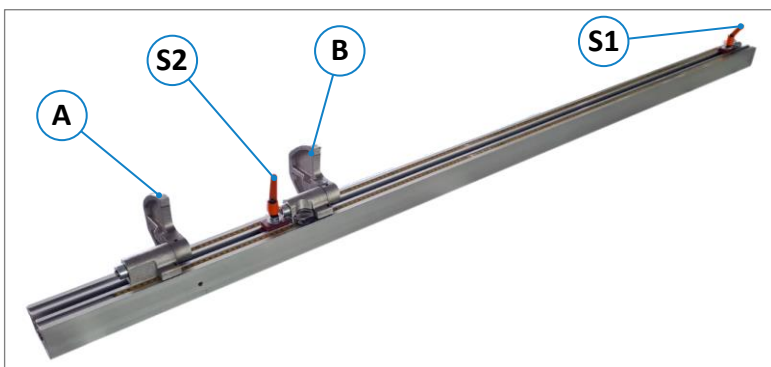
Figure 30 : guide télescopique
