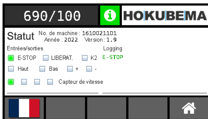
Figure 33 : fenêtre de statut
