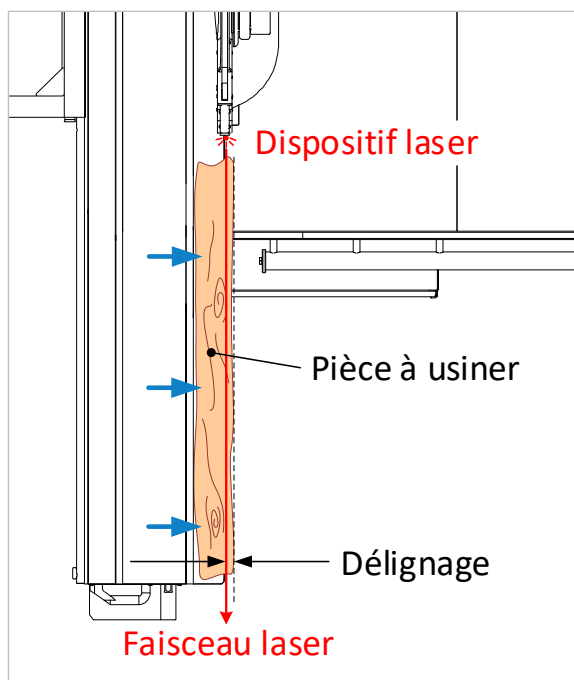
Figure 77 : délignage par faisceau laser
