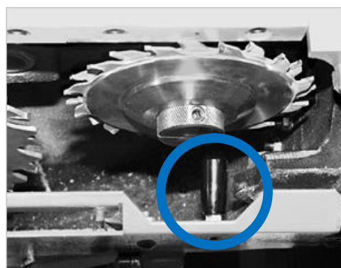
Figure 74 : cliquet d'arrêt du clapet à copeaux
