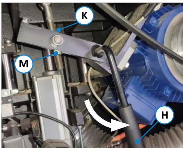
Figure 88 : tendre la courroie trapézoïdale
