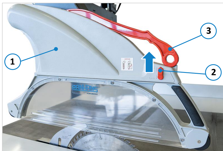
Figure 27 : monter le capot de protection
