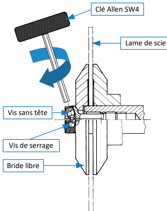
Figure 73 : bride de l'inciseur
