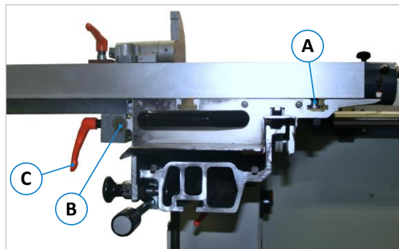
Figure 55 : structure du guide parallèle en option
