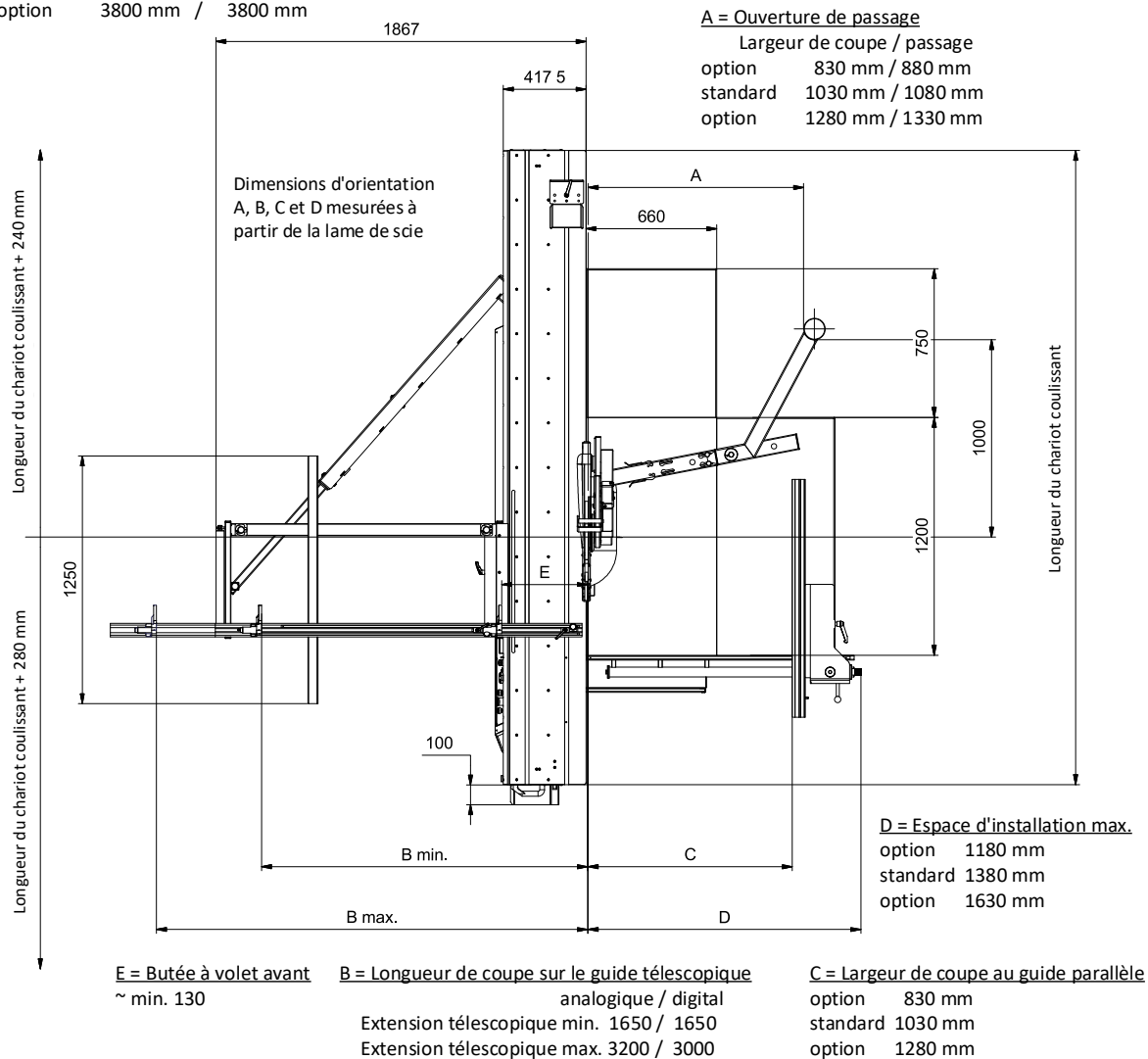
Figure 9 : dimensions (vue de dessus)
