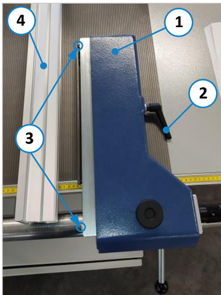
Figure 21 : monter le guide parallèle
