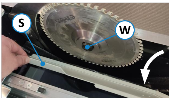
Figure 47 : rabattre le clapet à copeaux vers l'avant
