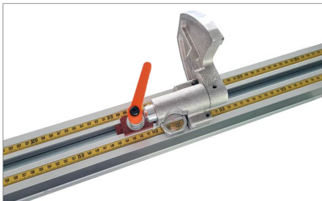
Figure 29 : butée à volet avec échelle de mesure et loupe
