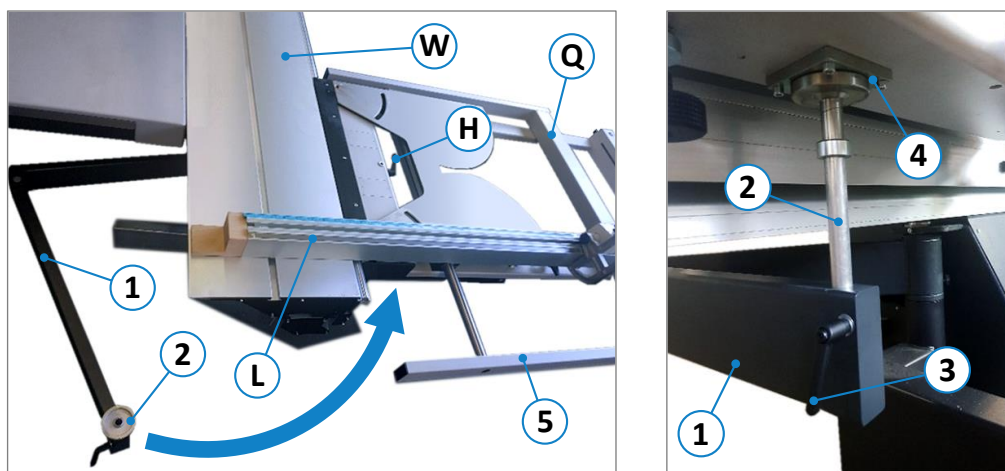
Figure 78 : positionner et monter le bras pivotant
