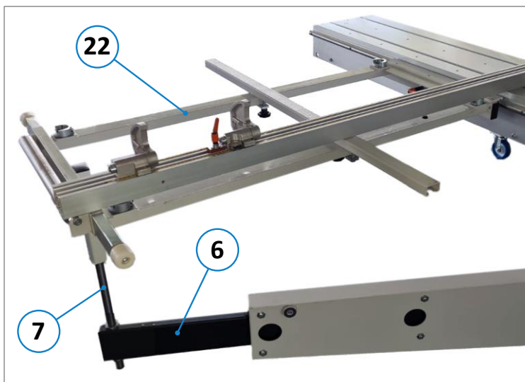
Figure 23 : montage du châssis à équarrir
