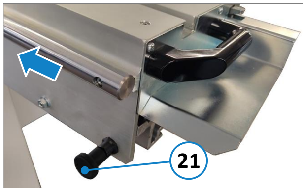
Figure 45 : blocage sur la table coulissante
