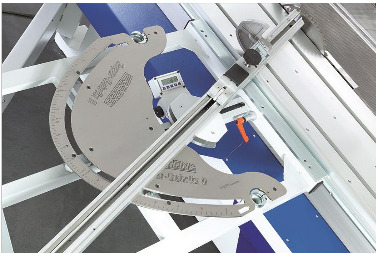
Figure 62 : guide à onglets et de longueur « SUPER-GEHRFIX II »
