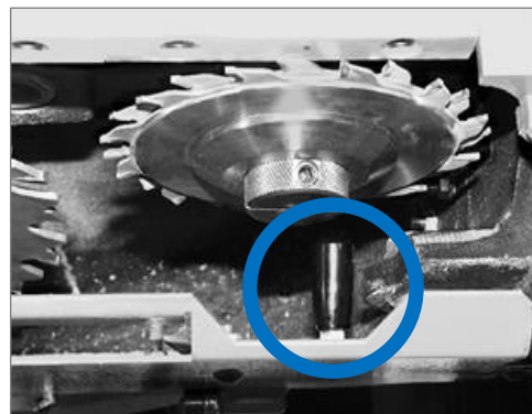
Abbildung 82: Sperrklinke Späneklappe
