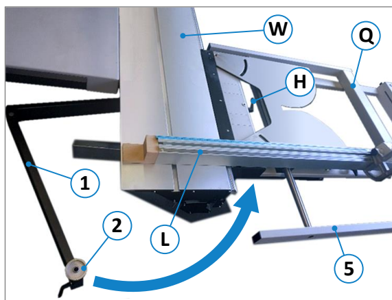
Abbildung 87: Wegschwenkarm positionieren & montieren
