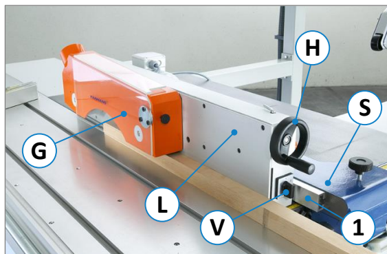
Abbildung 77: Vorschubapparat 76
