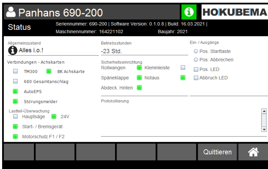
Abbildung 31: Statusanzeige
