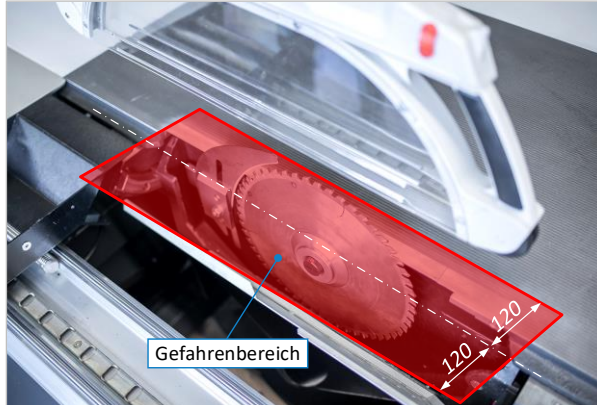
Abbildung 2: Gefahrenbereich Kreissägeblatt
