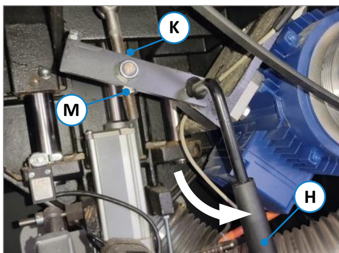
Abbildung 108: Keilriemenspannung
