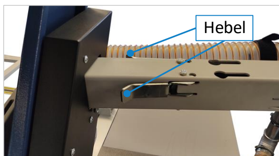
Abbildung 24: Schwenkarm für Schutzhaube
