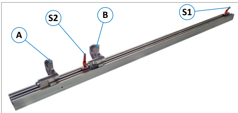
Abbildung 28: Längenanschlag Bedienelemente
