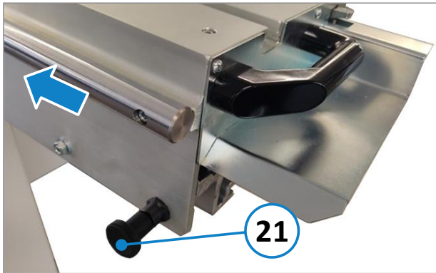
Abbildung 55: Fernarretierung am Rollwagen
