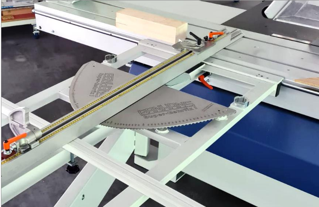
Abbildung 69: Super-Gehrfix I
