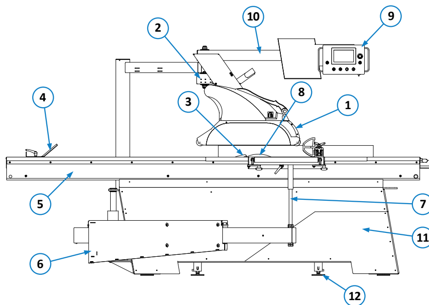
Abbildung 17: Komponenten / Bedienelemente - Vorderansicht
