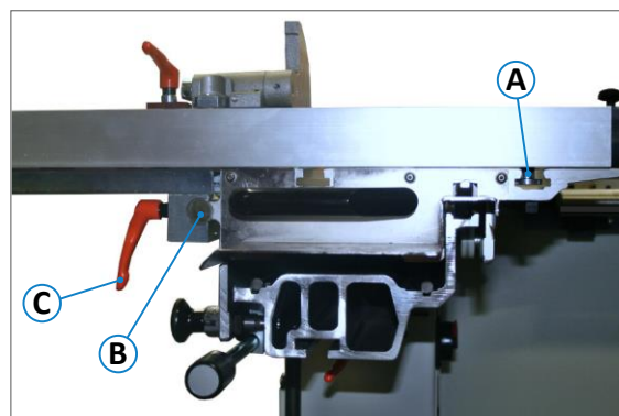
Abbildung 65: Aufbau - Parallelanschlag links v. Sägeblatt
