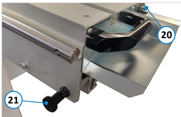
Abbildung 19: Rollwagen Bedienelemente
