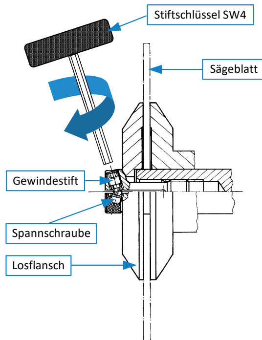
Abbildung 81: Sägeblattflansch der Vorritzsäge
