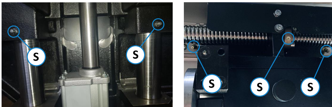
Abbildung 109: Schmierstellen an der Höhenverstellung
