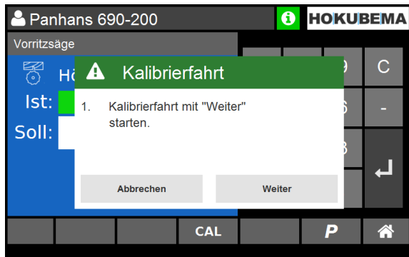
Abbildung 41: Vorritzsäge kalibrieren
