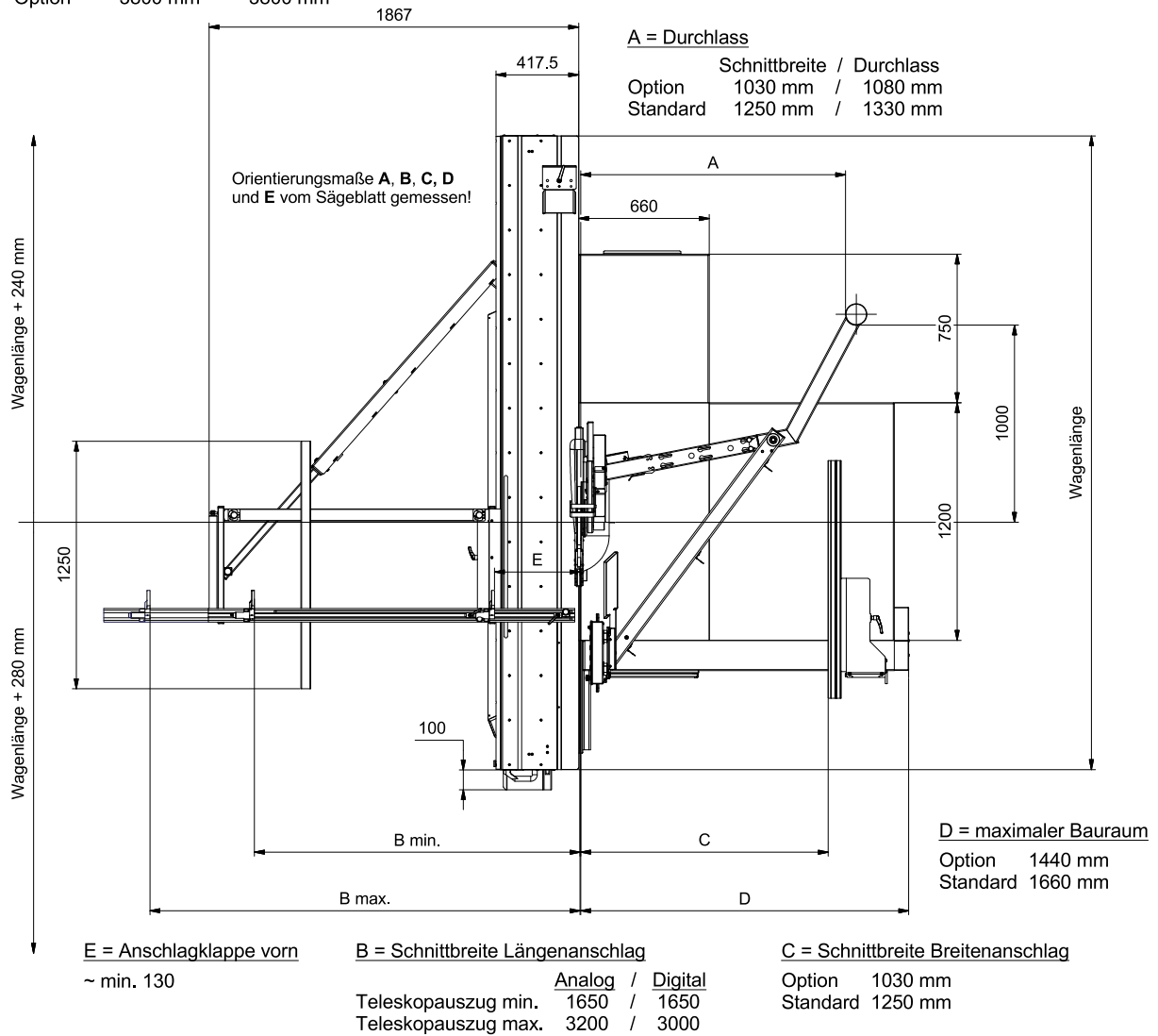
Abbildung 9: Abmessungen (Draufsicht)
