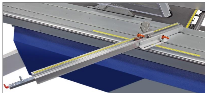
Abbildung 76: Standard-Gehrungsanschlag
