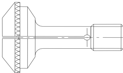
Abbildung 80: Quickstep Schnellspannschraube
