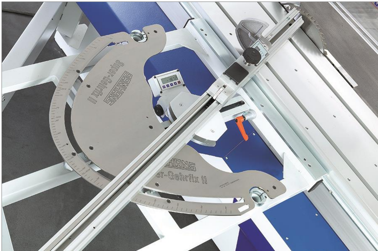
Abbildung 72: Super-Gehrfix II
