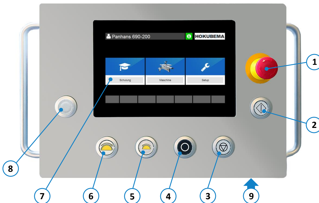
Abbildung 26: Bedienelemente
