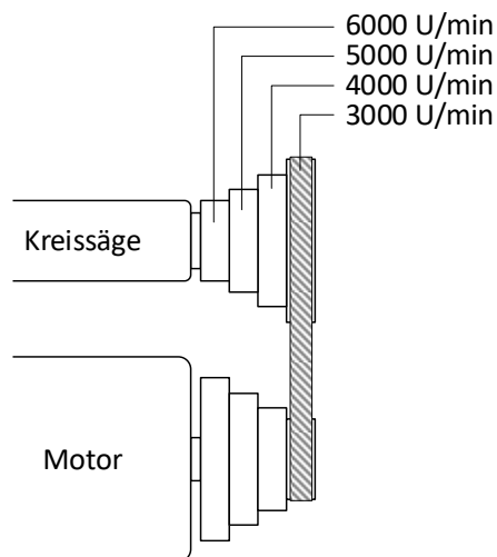
Abbildung 44: Drehzahlschema
