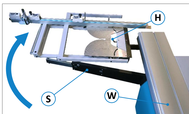
Abbildung 88: Querschlitten wegschwenken
