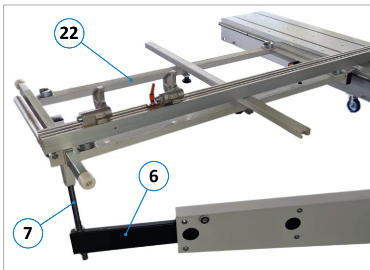
Abbildung 21: Querschlitten Montage
