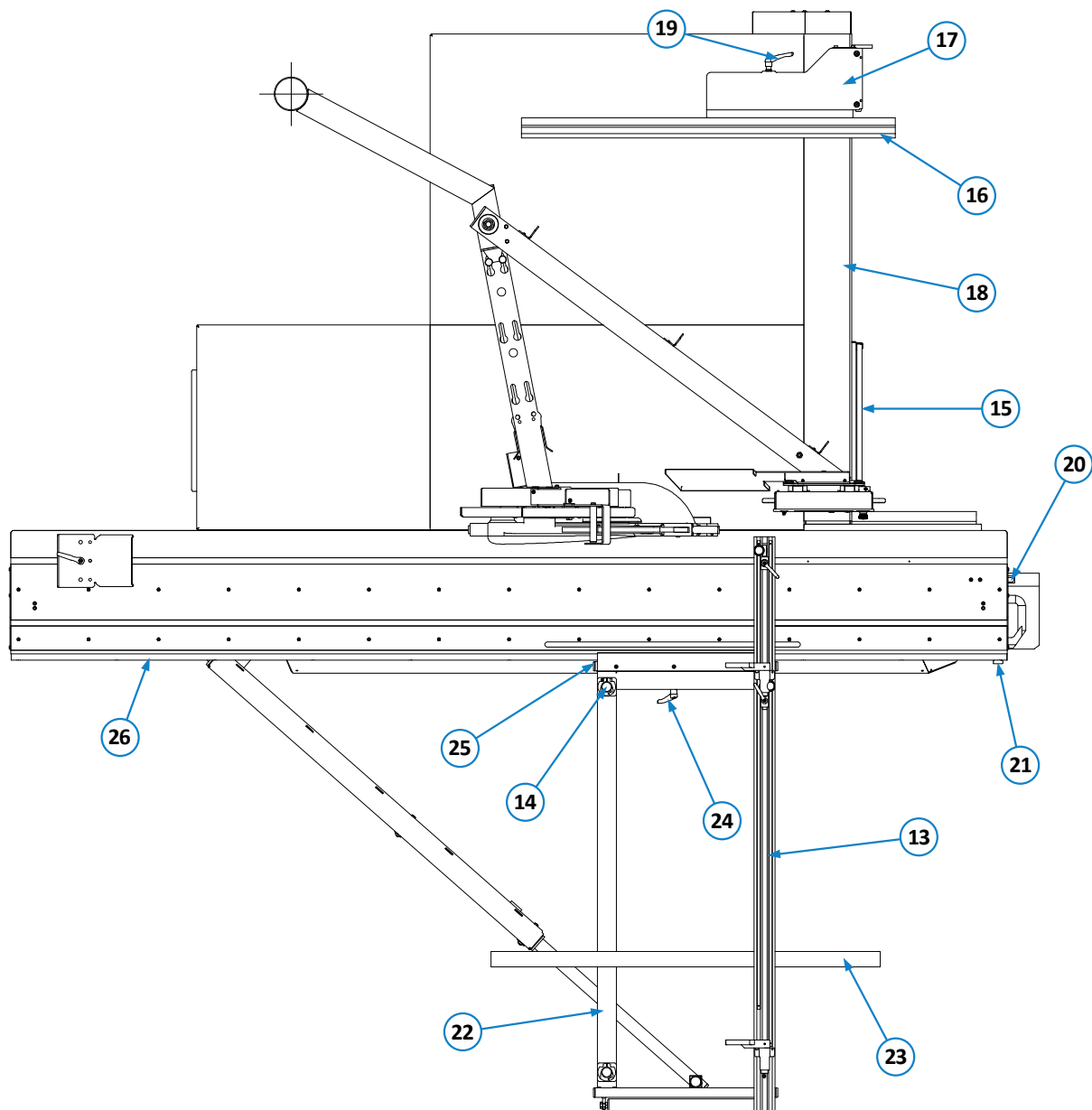
Abbildung 18: Komponenten / Bedienelemente – Draufsicht
