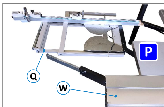
Abbildung 89: Endgültige Parkposition
