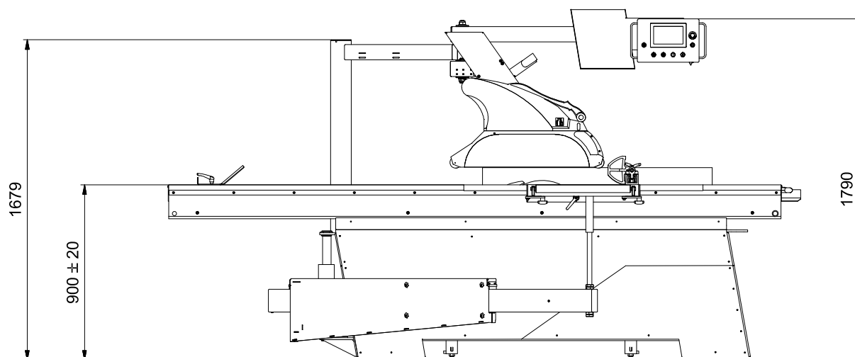
Abbildung 8: Abmessungen (Draufsicht)
