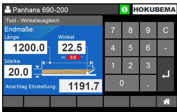
Abbildung 48: Tool für Winkelausgleich
