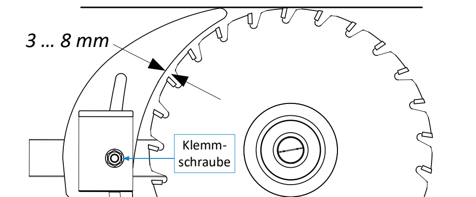
Abbildung 59: Spaltkeileinstellung (Symbolische Darstellung)
