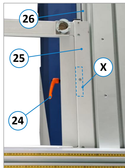
Abbildung 22: Querschlitten Klemmung
