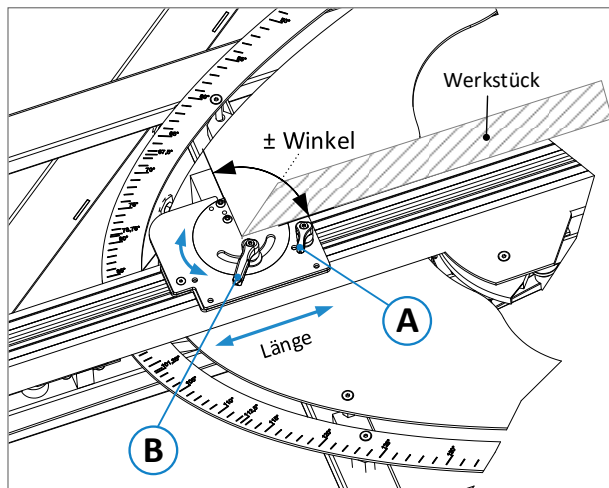
Abbildung 75: Bedienung des Gehrungs-Hilfsanschlages
