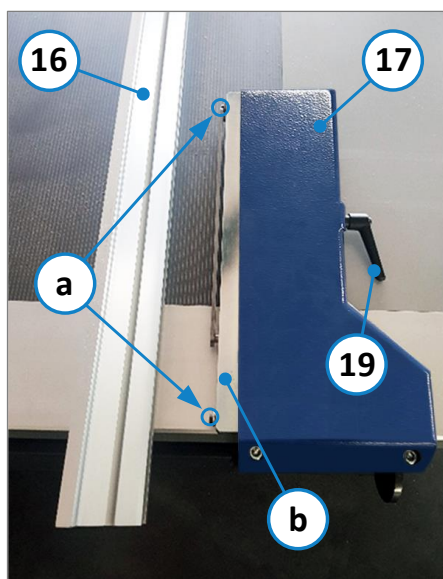
Abbildung 20: Parallelanschlag montieren
