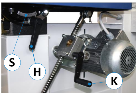
Abbildung 41: Tischneigung einstellen
