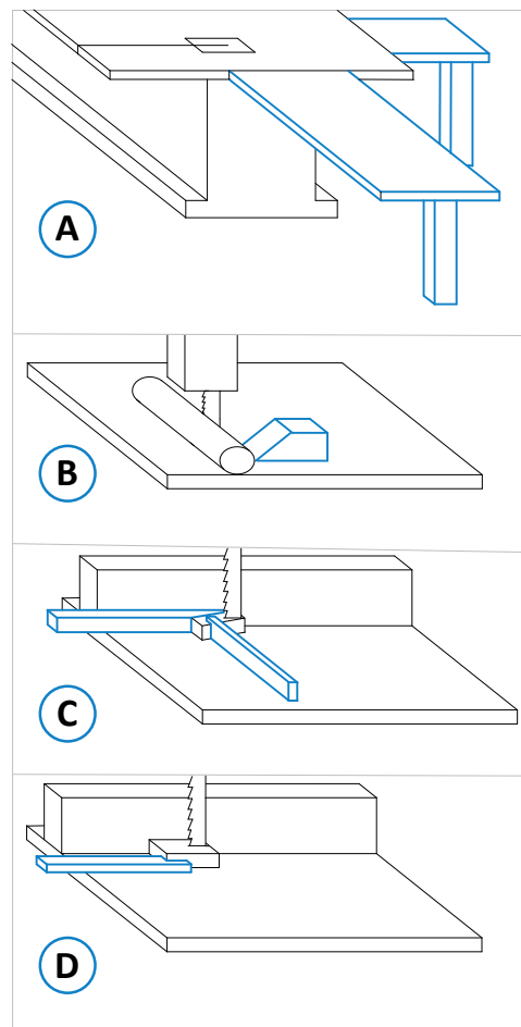
Abbildung 38: Tischverlängerungen und Hilfsmittel
