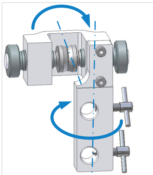
Abbildung 32: Führung unten auf links umbauen
