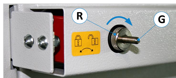
Abbildung 23: Sicherheitsschalter - Türe entriegelt
