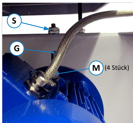
Abbildung 51: Keilriemen nachspannen
