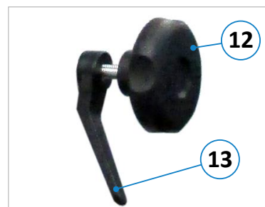
Abbildung 26: Bandsägeradverstellung
