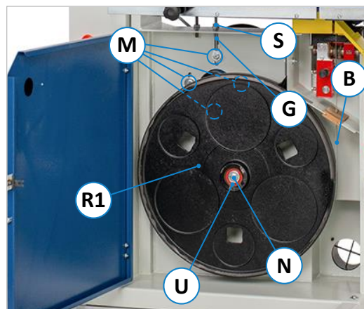
Abbildung 52: Keilriemen auswechseln
