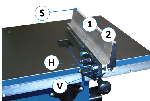
Abbildung 36: Anschlag für Linkshänder umbauen
