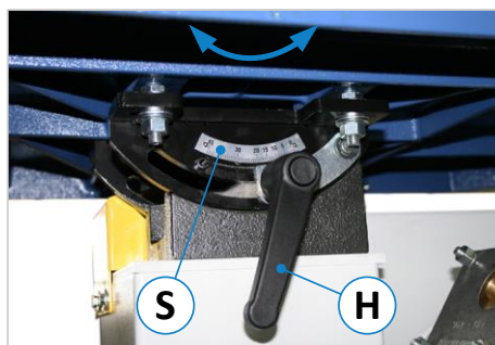
Abbildung 28: Tischneigung einstellen
