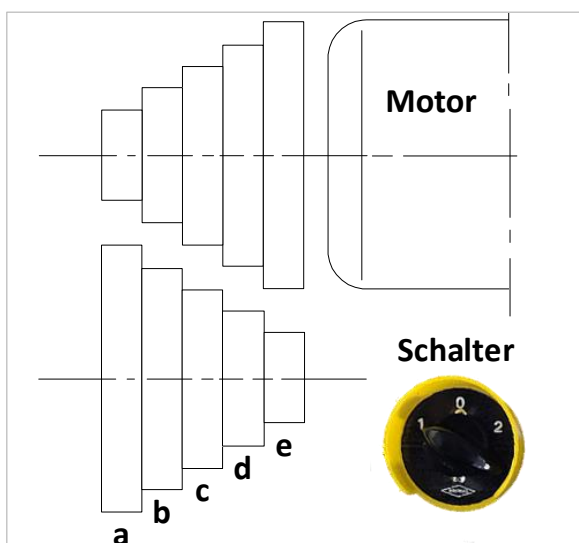
Abbildung 79: Riemenlagen für Vorschubgeschwindigkeit
