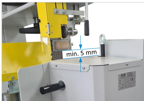
Abbildung 66: Kollisionsgefahr am Sägeblattschutz
