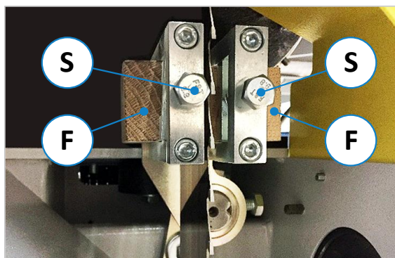
Abbildung 62: Untere Sägeblattführung
