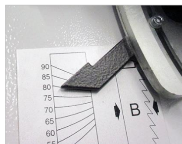
Abbildung 58: Blattspannungsanzeige
