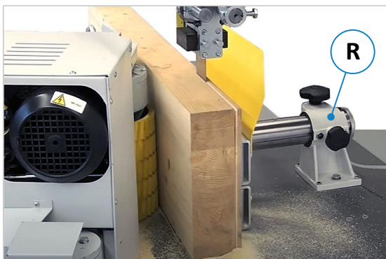
Abbildung 70: Rollenanschlag und Vorschub im Einsatz
