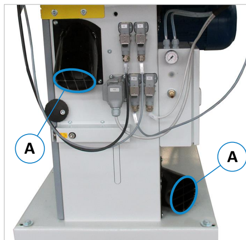
Abbildung 26: Absauganschlüsse
