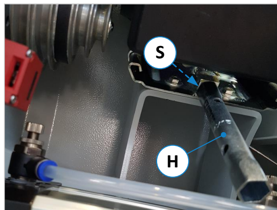
Abbildung 78: Riemenspannung lösen
