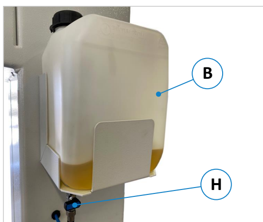
Abbildung 83: Schmierstoffbehälter mit Absperrhahn
