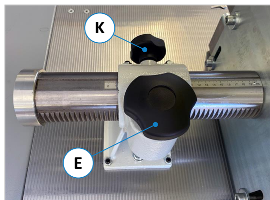
Abbildung 73: Einstellung des Schnittmaßes
