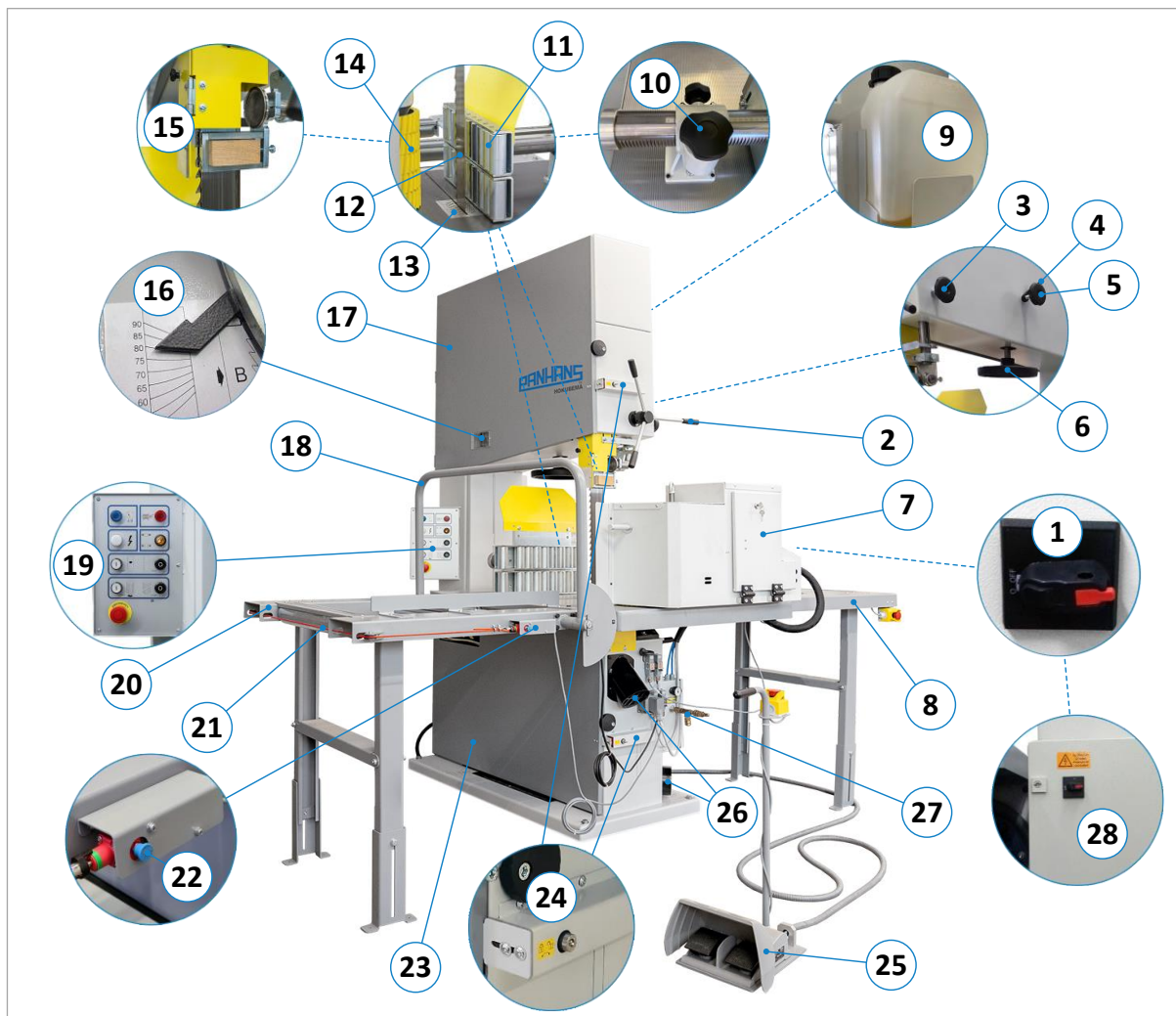
Abbildung 28: Komponenten / Bedienelemente
