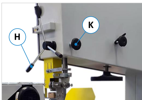
Abbildung 63: Höhenverstellhebel
