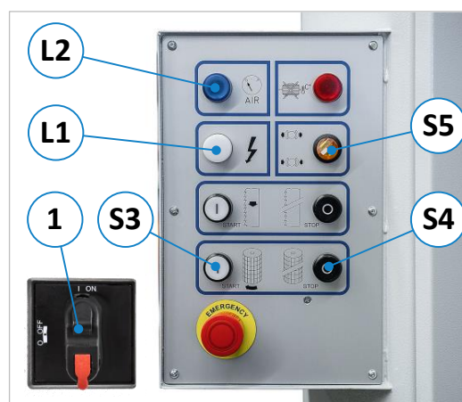
Abbildung 76: Bedienschaltpult für den Vorschubantrieb
