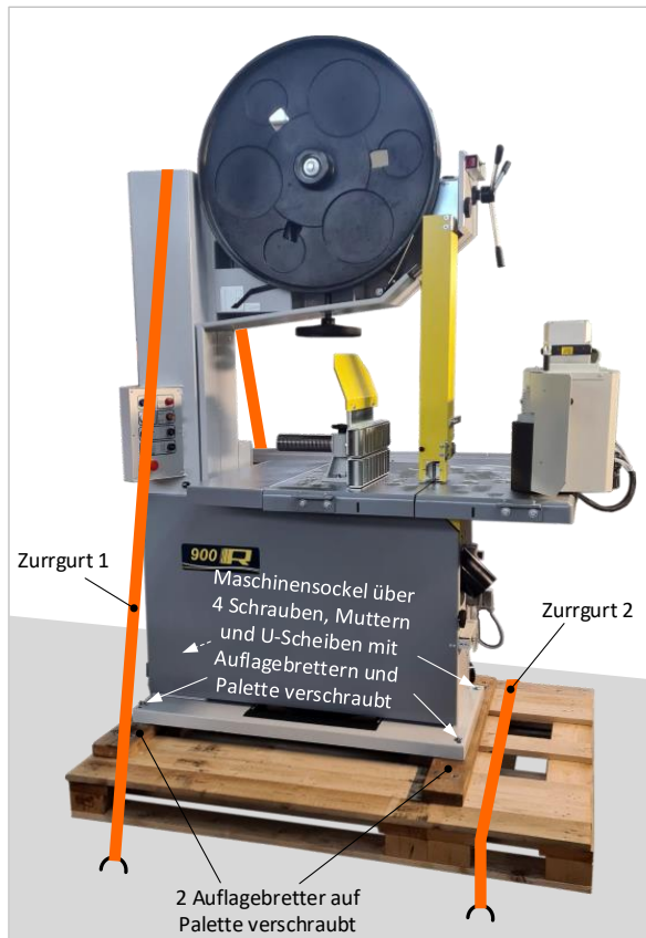
Abbildung 12: Maschine auf Palette verzurren
