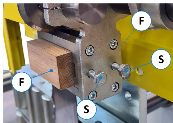
Abbildung 65: Seitenführungen einstellen
