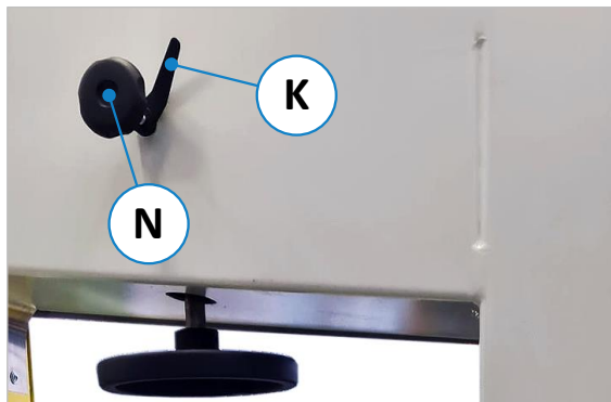
Abbildung 60: Sägeblattneigung korrigieren
