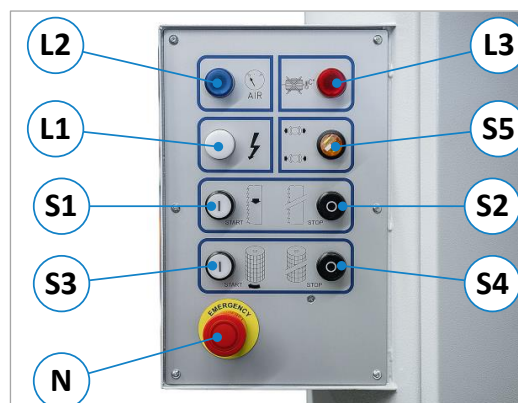
Abbildung 42: Maschine ein- /ausschalten
