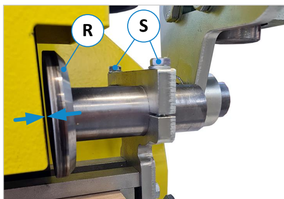
Abbildung 64: Rückenrolle einstellen
