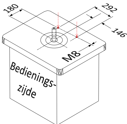
Figuur 13: Draadgaten boren
