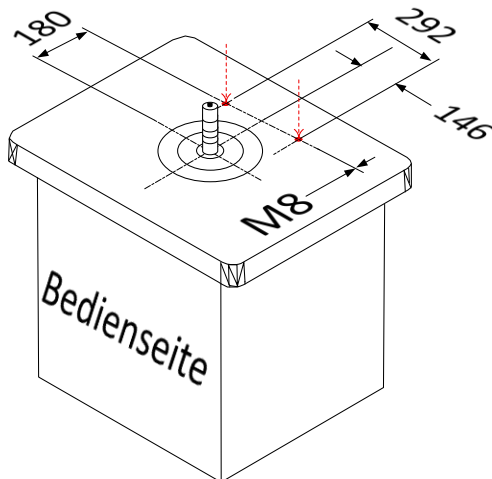
Abbildung 1: Gewindebohrungen einbringen
