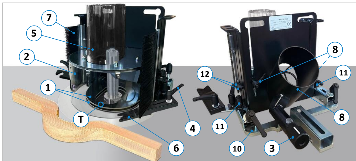
Figuur 15: Bedieningselementen van de bogenfreesaanslag KOALA 1637
