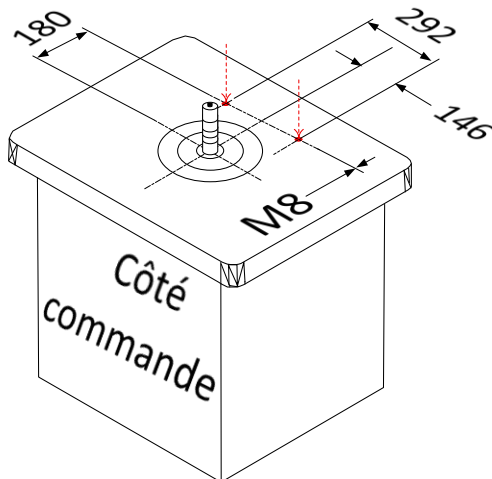
Figure 9 : Réaliser des taraudages
