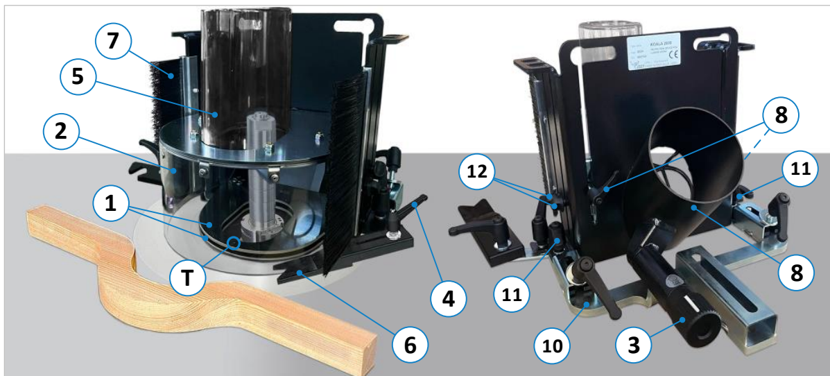
Figure 11 : Éléments de commande du guide de fraisage courbe KOALA 1637
