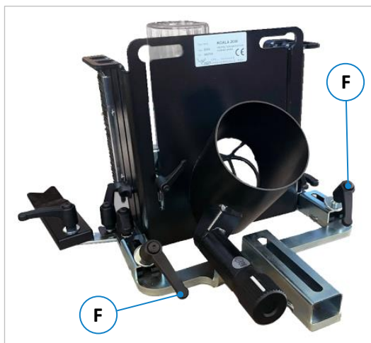
Figuur 14: Bevestiging op de freestafel
