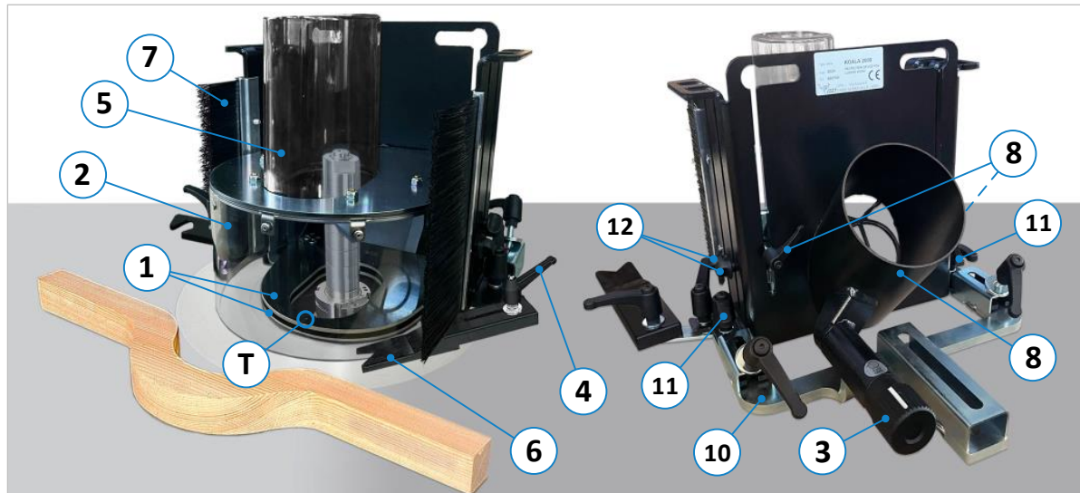
Abbildung 3: Bedienelemente des Bogenfräsanschlags KOALA 1637
