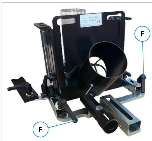
Abbildung 2: Befestigung auf dem Frästisch
