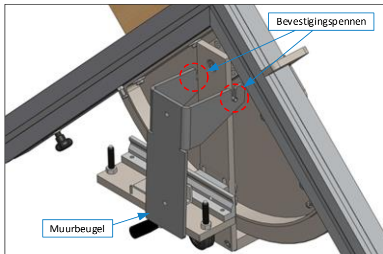
Figuur 13: DSG-A muurbeugel
