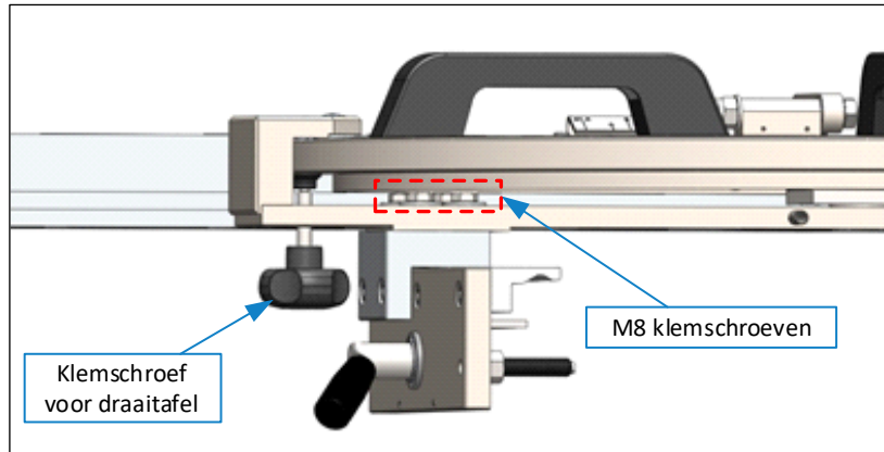
Figuur 4: DSG-A aanpassen (1)
