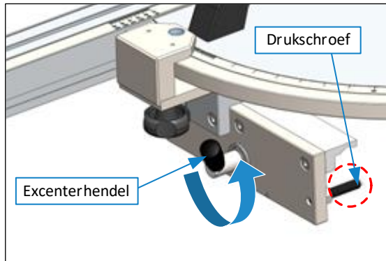
Figuur 2: Plaats DSG-A op loopwagen
