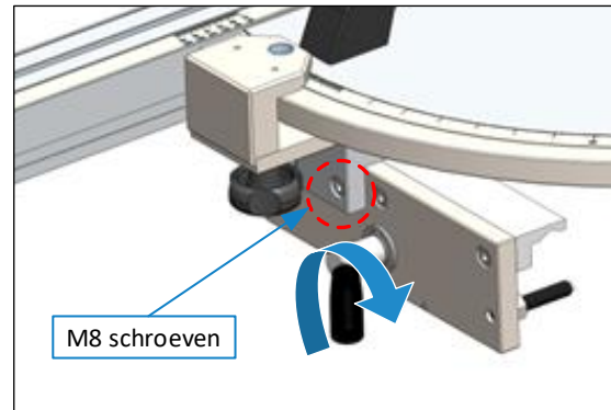
Figuur 3: DSG-A op loopwagen vastzetten
