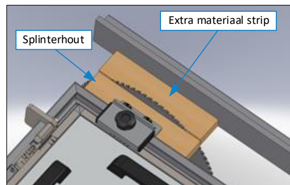
Figuur 6: DSG-A aanpassen (3)
