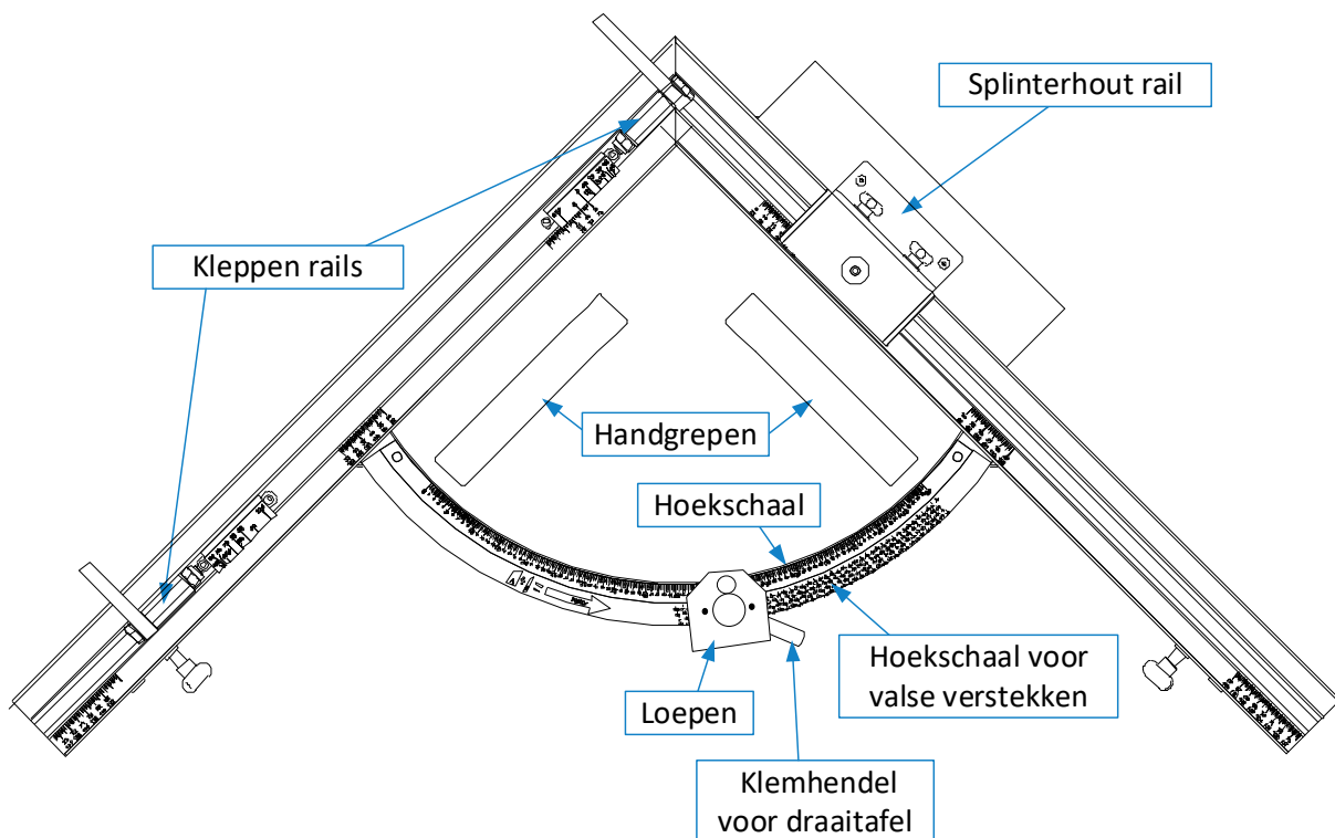
Figuur 1: Bedieningselementen DSG-A
