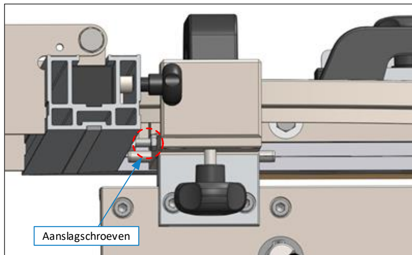
Figuur 5: DSG-A aanpassen (2)
