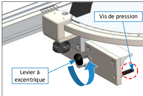
Figure 2 : placer le DSG-D sur la table coulissante
