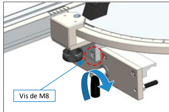
Figure 3 : fixer le DSG-D sur la table coulissante
