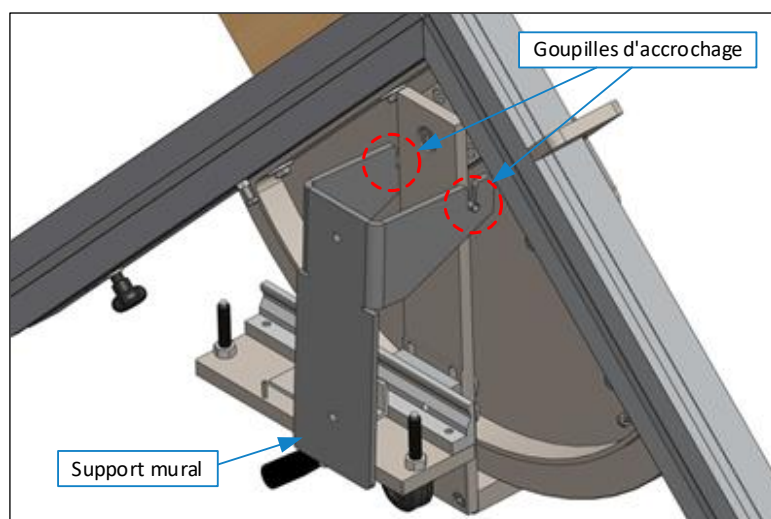
Figure 15 : support mural pour DSG-D
