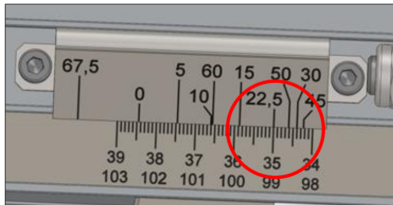
Figure 8 : exemple de réglage DSG-D
