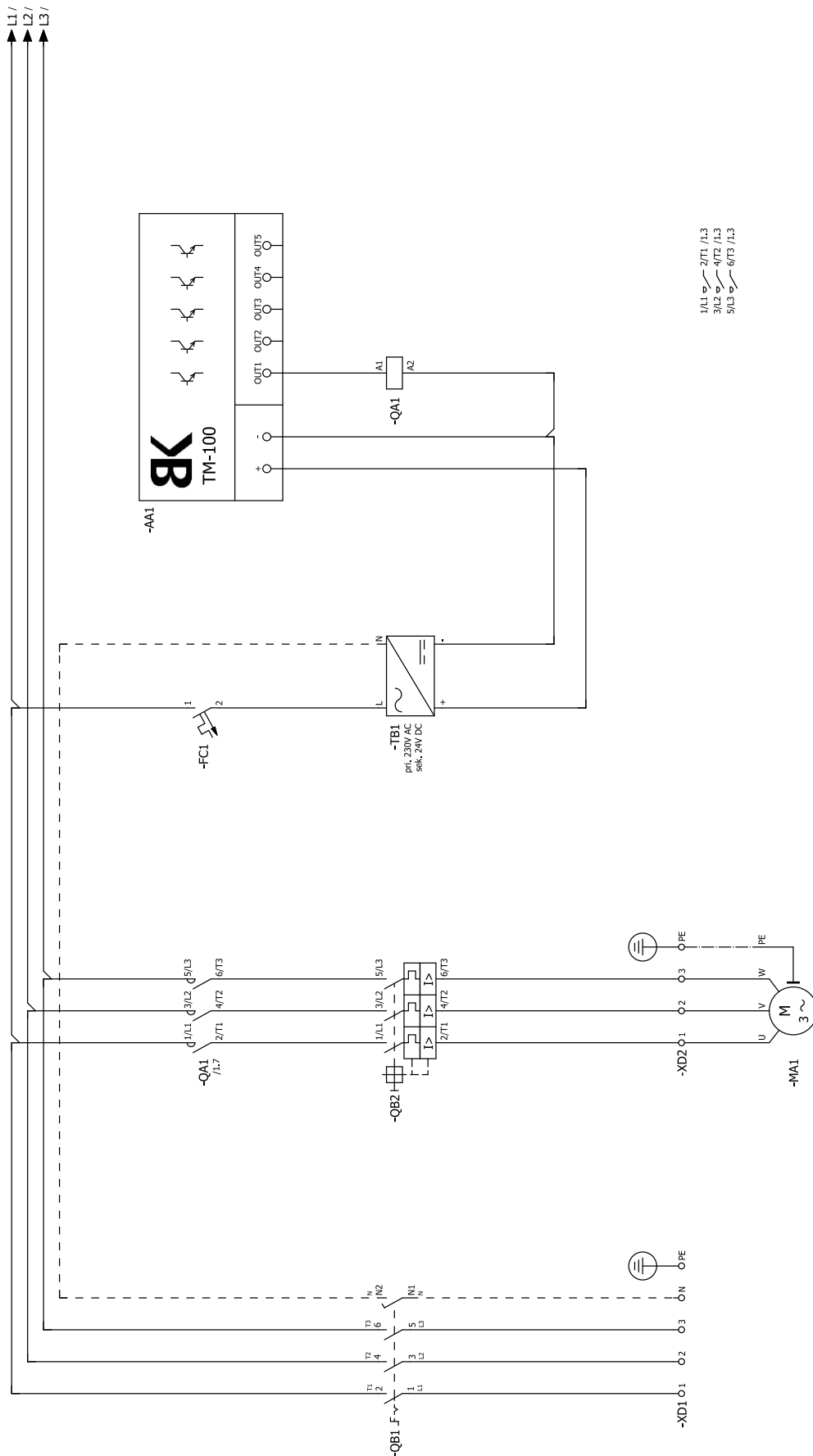
Abbildung 6: Schaltplan TM-100
