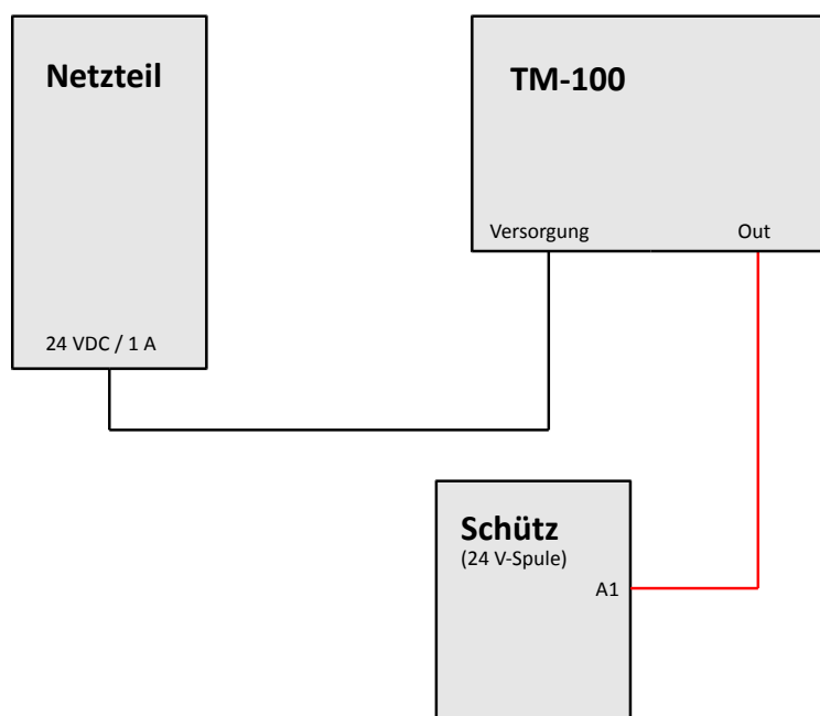
Abbildung 5: Blockschaltbild
