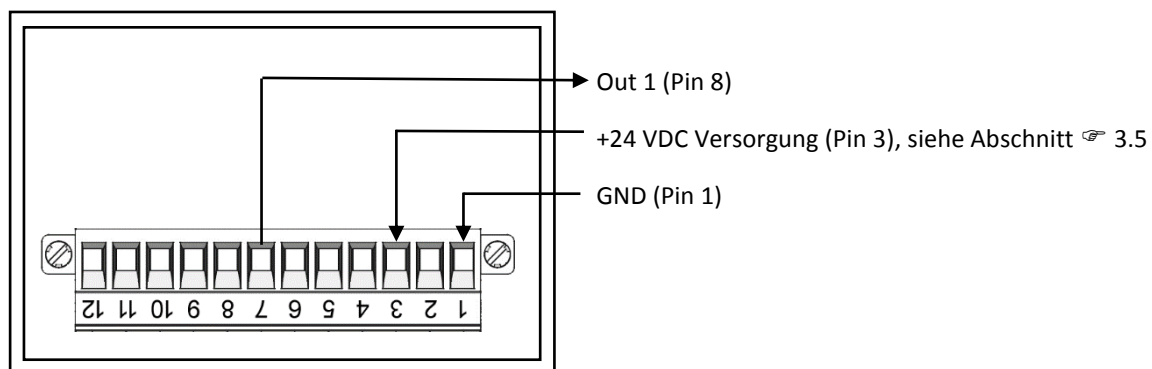
Abbildung 2: Beispiel-Verdrahtung „Out 1“ (Pin 8)
