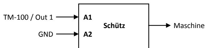
Abbildung 4: Externer Schütz mit 24 VDC Spule
